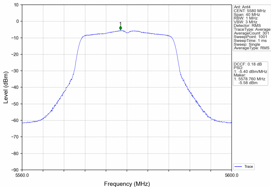
802.11n(HT20)_MCH_5580MHz_Ant4_NTNV
