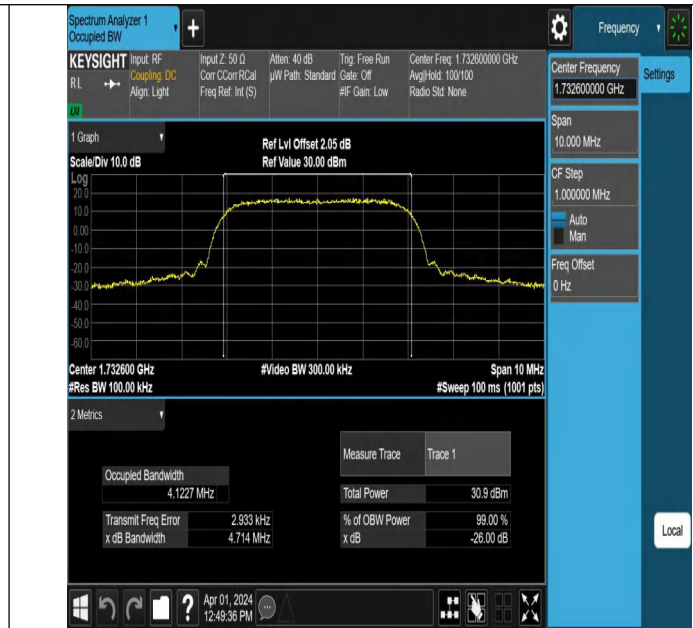
Band4-1413-5-PASS
