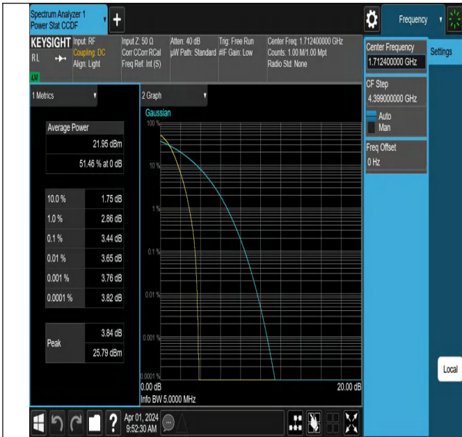
Band4-1312-1-PASS
