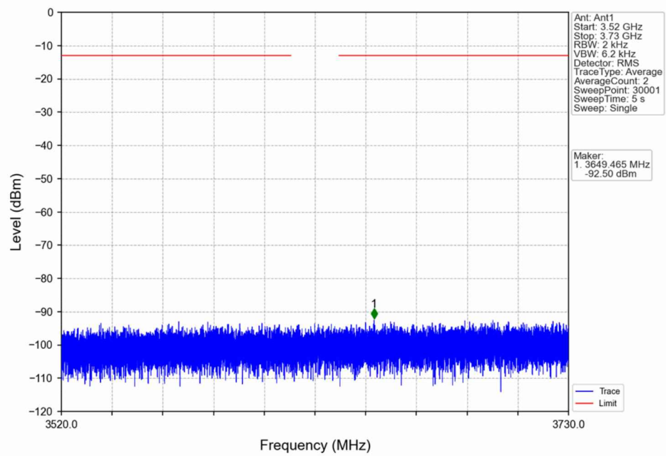
n48_30kHz_SISO_NTNV_20MHz_CP-OFDM QPSK_3624.99MHz_Edge_1RB_Left
