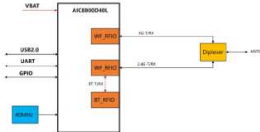
SKI.WB800D80U.2_D40L单天线配置系统框图
