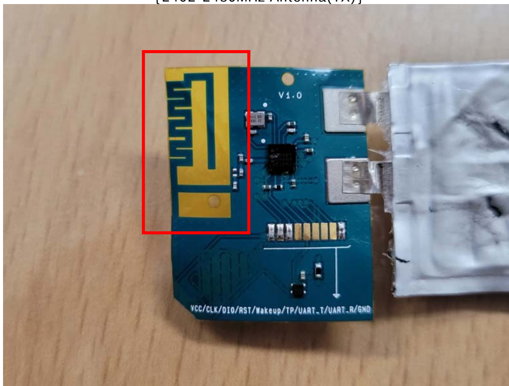
{ 2402-2480MHz Antenna(TX) }
