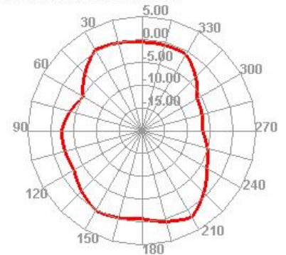
2090.000MHz E2
