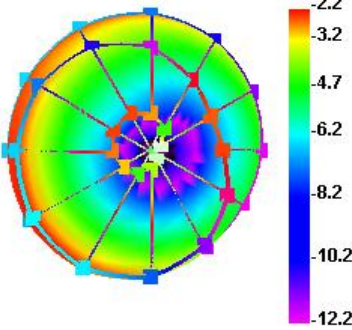
870.000MHz
