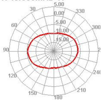
1740.000MHz H
