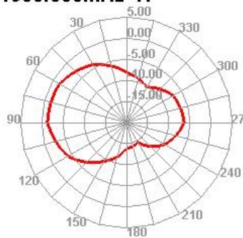
1930.000MHz H
