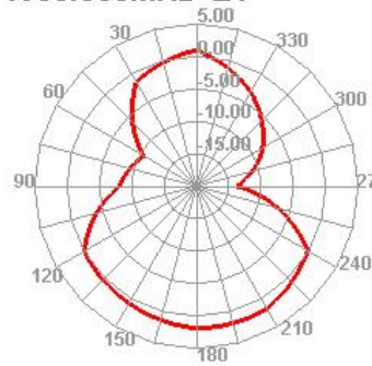
1930.000MHz E1
