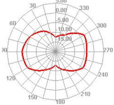
1740.000MHz E2
