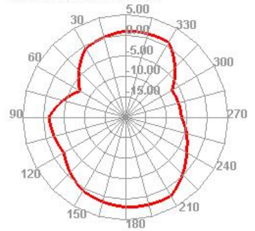
1930.000MHz E2
