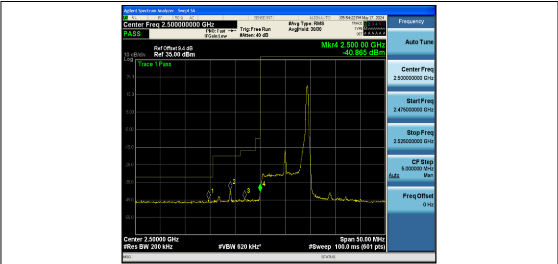
Band7-10MHz-QPSK-20800-50RB#0
