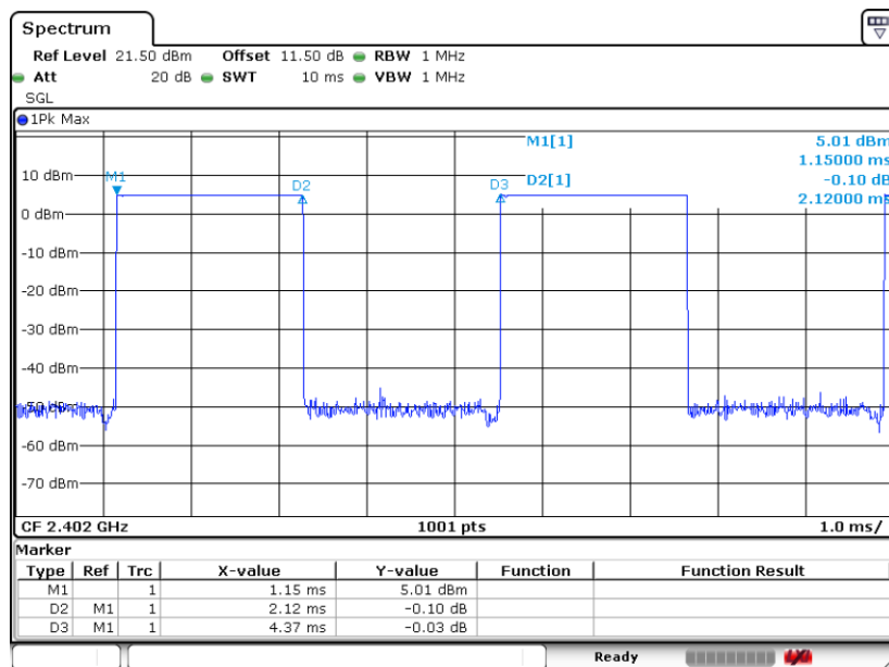
BLE(CH0-39) 1Mbps
