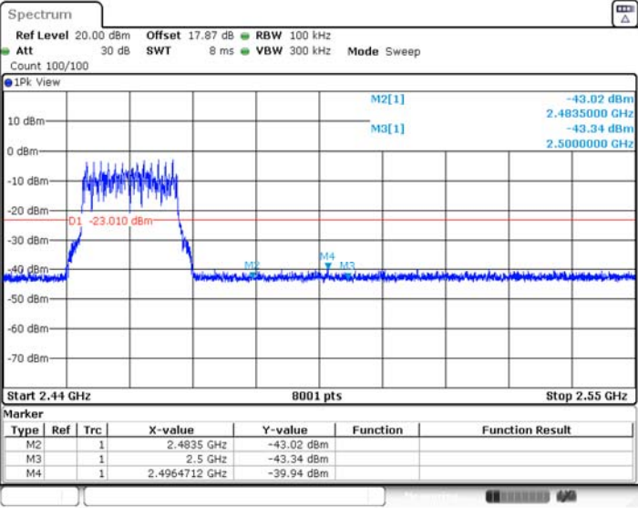
11N20MIMO_Ant2_High_2462
