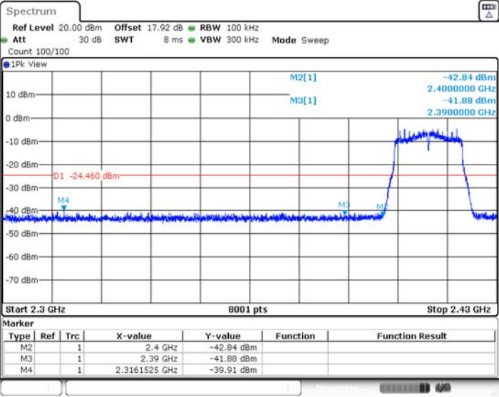
11N20MIMO_Ant2_Low_2412
