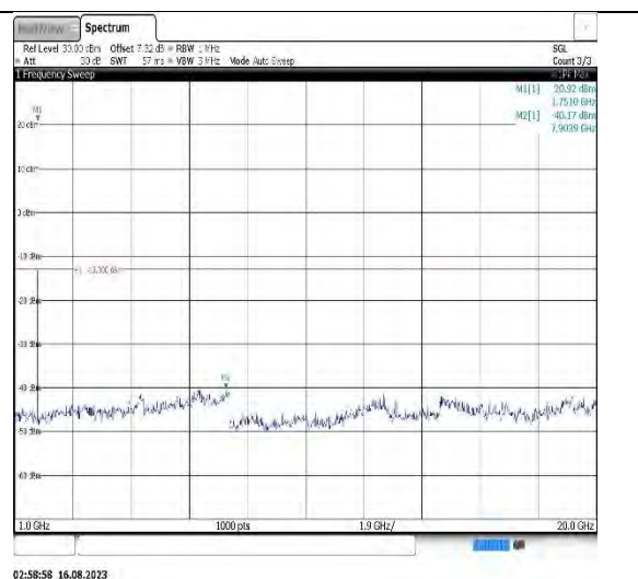
Band4-5MHz-QPSK-19975-1RB#0-Range2:1000~20000MHz
