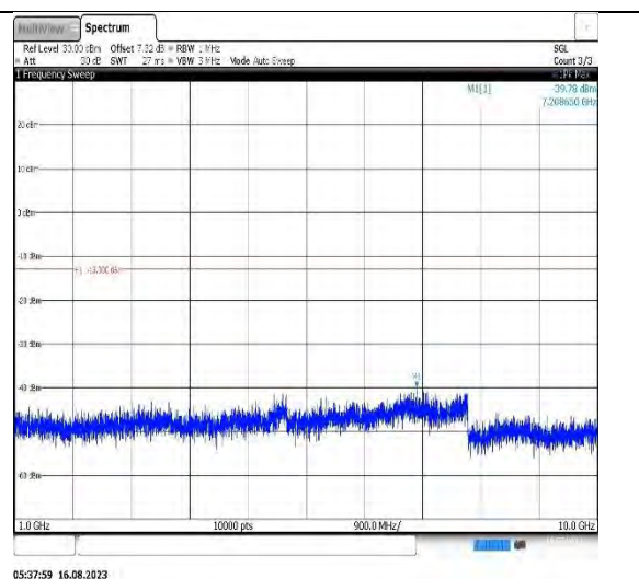
Band5-3MHz-QPSK-20415-1RB#0- Range2:1000~10000MHz
