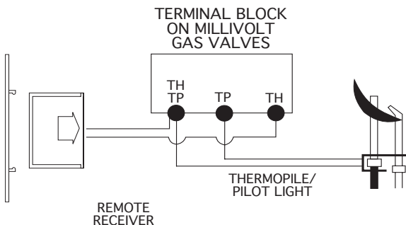
Fig. 24 Millivolt wiring.
