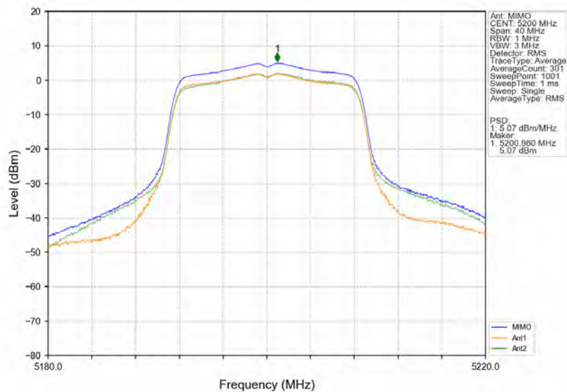
802.11a MCH 5200MHz MIMO NTN
