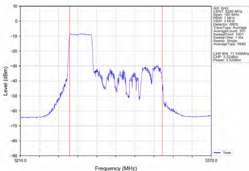
802.11ax(HE80) MCH 5290MHz RU242 Left Ant2 NTN
