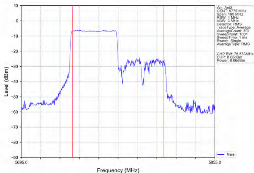
802.11ax(HE80) MCH 5775MHz RU484 Left Ant2 NTN
