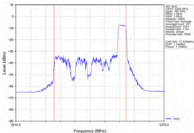
802.11ax(HE80) MCH 5290MHz RU106 Right Ant2 NTVN
