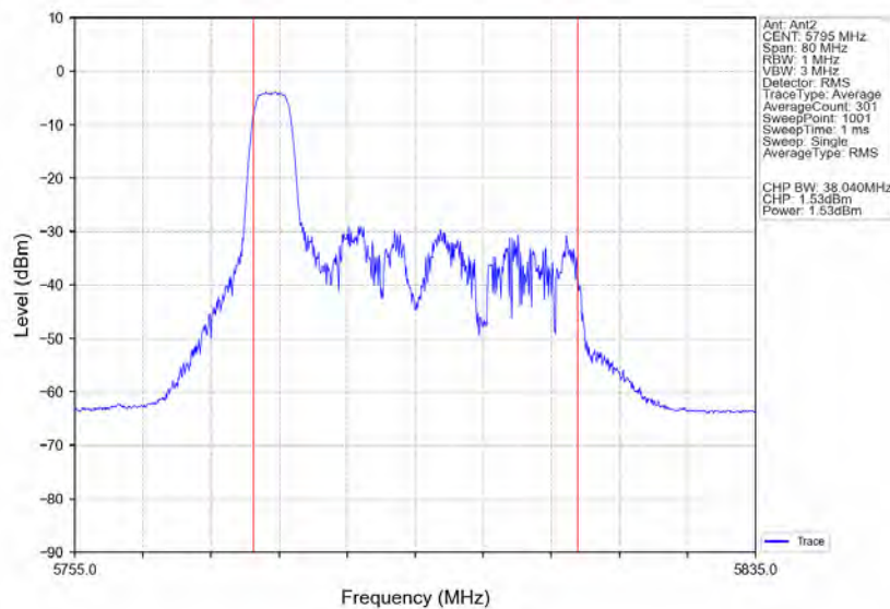
802.11ax(HE40) HCH 5795MHz RU52 Left Ant2 NTN
