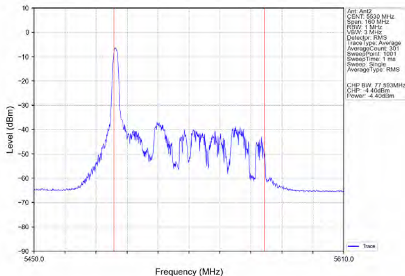
802.11ax(HE80) LCH 5530MHz RU26 Left Ant2 NTN
