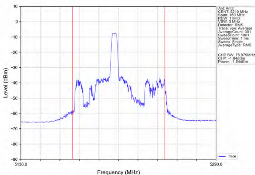
802.11ax(HE80) MCH_5210MHz RU52_Mid_Ant2_NTNV
