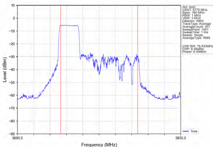
802.11ax(HE80) MCH 5775MHz RU242 Left Ant2 NTNv
