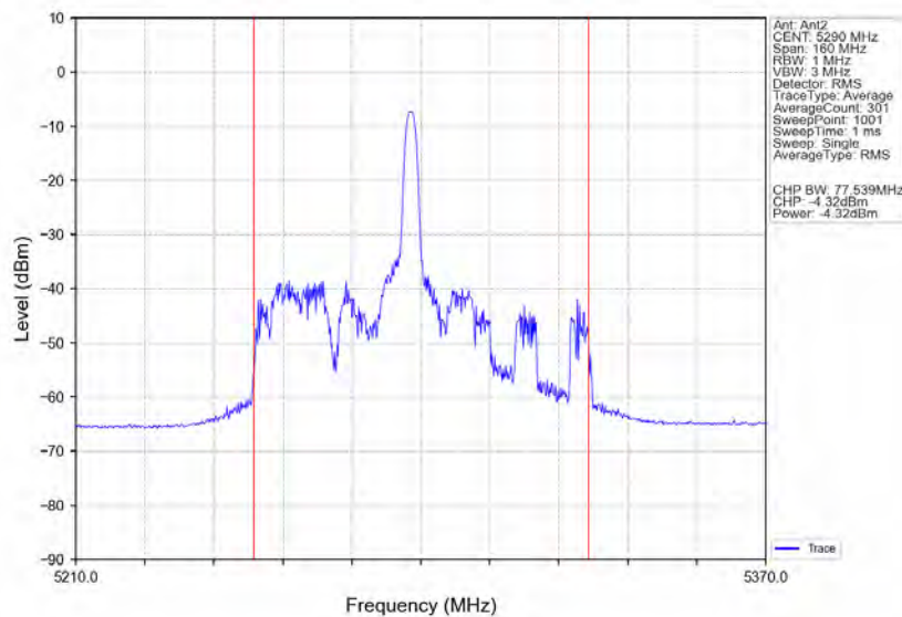
802.11ax(HE80) MCH 5290MHz RU26 Mid Ant2 NTN
