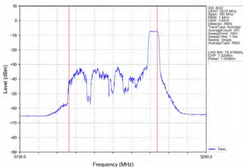
802.11ax(HE80) MCH 5210MHz RU106 Right Ant2 NTVN
