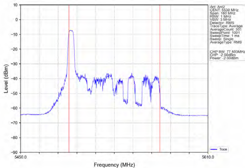
802.11ax(HE80) LCH 5530MHz RU52 Left Ant2 NTN
