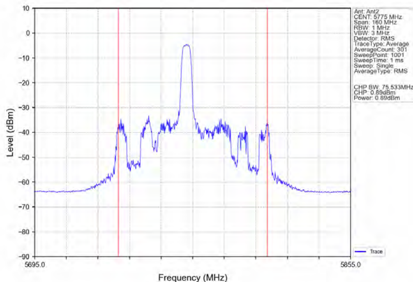
802.11ax(HE80) MCH_5775MHz RU52_Mid_Ant2_NTNV
