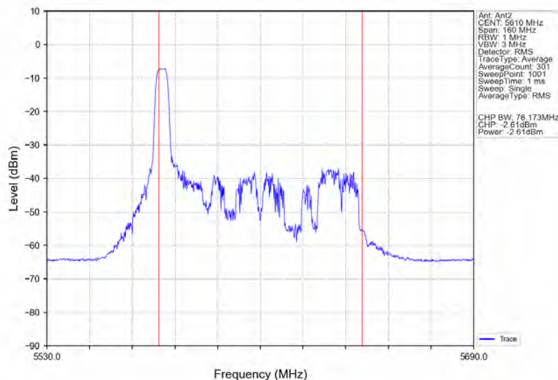
802.11ax(HE80) HCH 5610MHz RU52 Left Ant2 NTN
