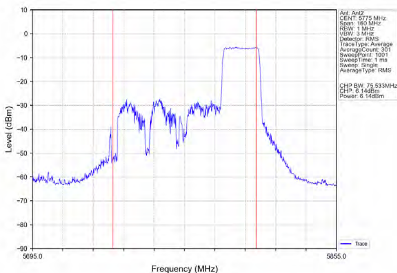
802.11ax(HE80) MCH_5775MHz RU242 Right Ant2 NTVN
