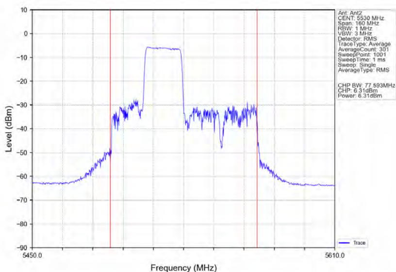
802.11ax(HE80) LCH 5530MHz RU242 Mid Ant2 NTNv
