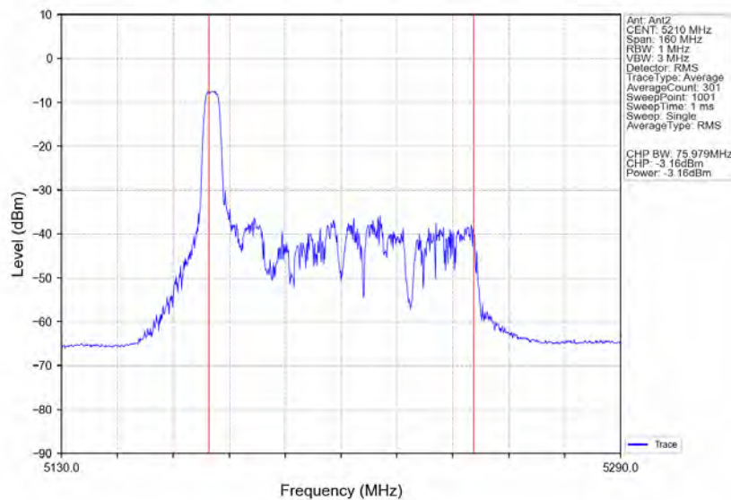
802.11ax(HE80) MCH_5210MHz RU52 Left Ant2 NTN
