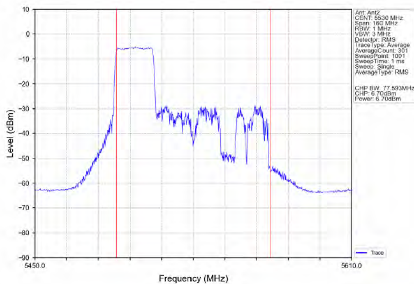
802.11ax(HE80) LCH 5530MHz RU242 Left Ant2 NTNv
