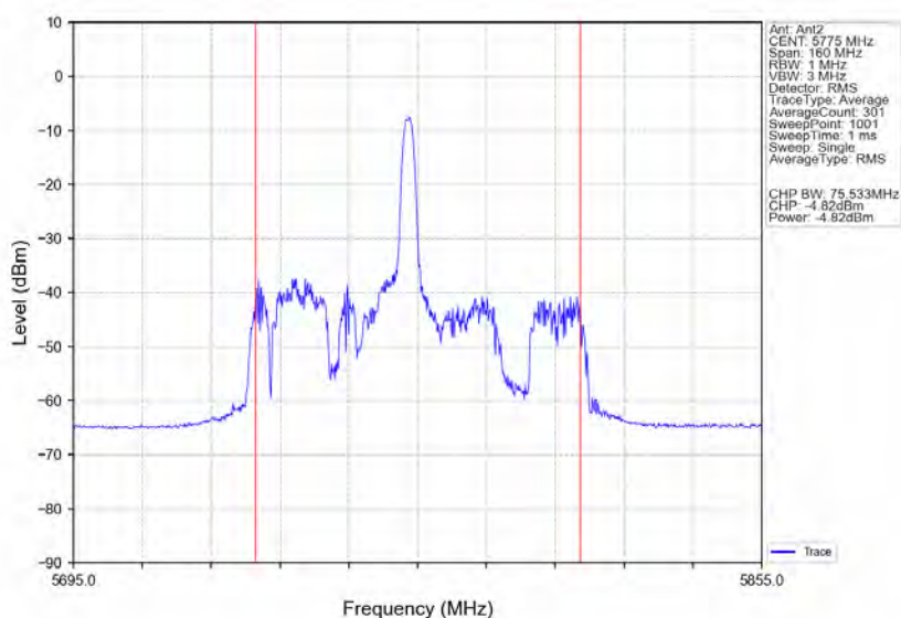
802.11ax(HE80) MCH_5775MHz RU26_Mid_Ant2_NTNV
