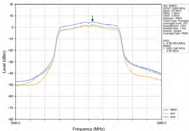
802.11a LCH 5260MHz MIMO NTN
