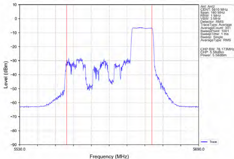
802.11ax(HE80) HCH 5610MHz RU242 Right Ant2 NTVN
