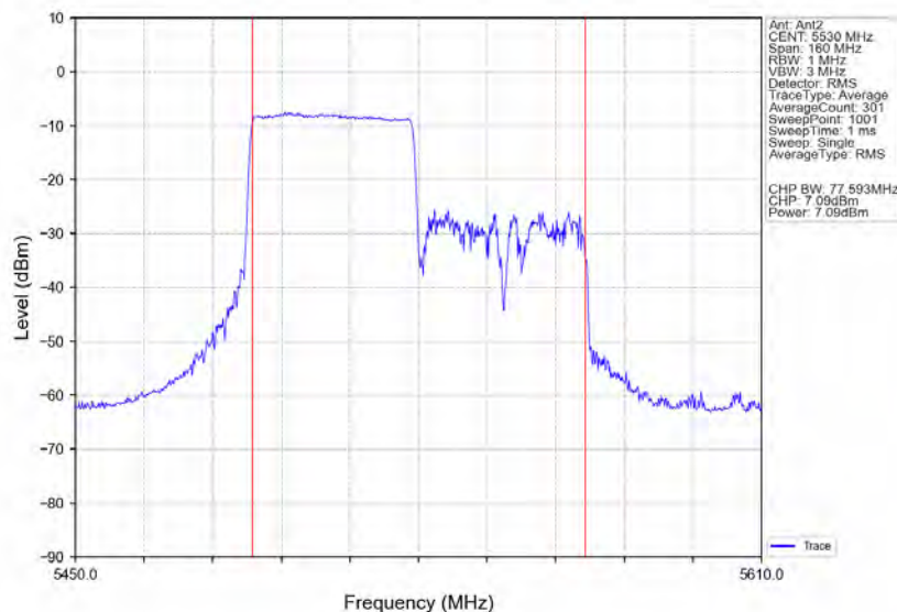
802.11ax(HE80) LCH 5530MHz RU484 Left Ant2 NTN
