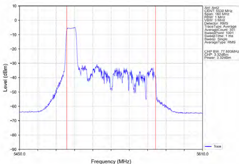
802.11ax(HE80) LCH 5530MHz RU106 Left Ant2 NTNv
