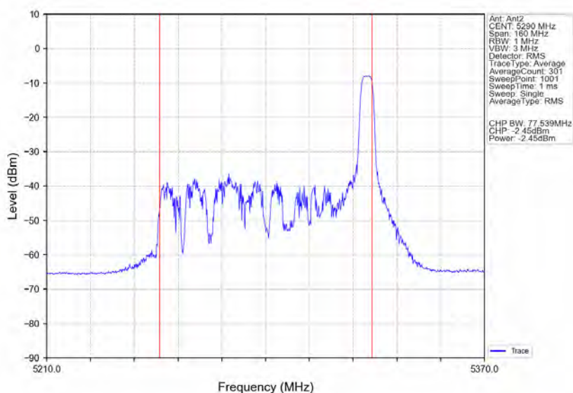
802.11ax(HE80) MCH 5290MHz RU52 Right Ant2 NTN
