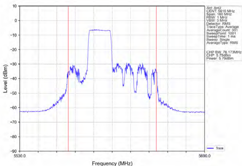
802.11ax(HE80) HCH 5610MHz RU242 Mid Ant2 NTNv
