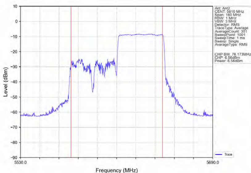
802.11ax(HE80) HCH 5610MHz RU484 Right Ant2 NTVN
