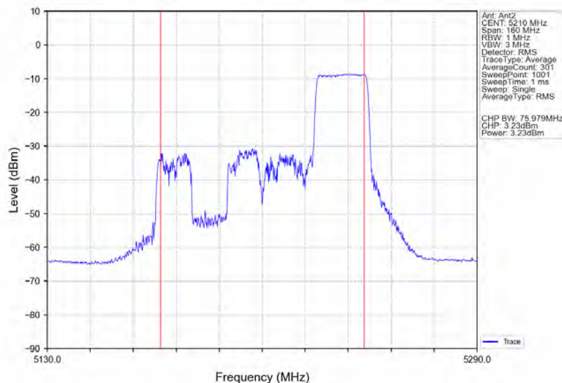
802.11ax(HE80) MCH_5210MHz RU242 Right Ant2 NTVN
