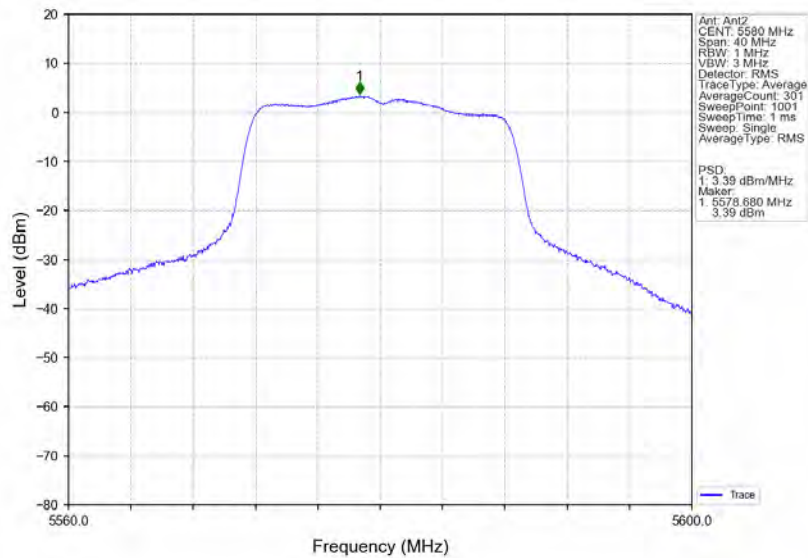
802.11a MCH 5580MHz MIMO NTN
