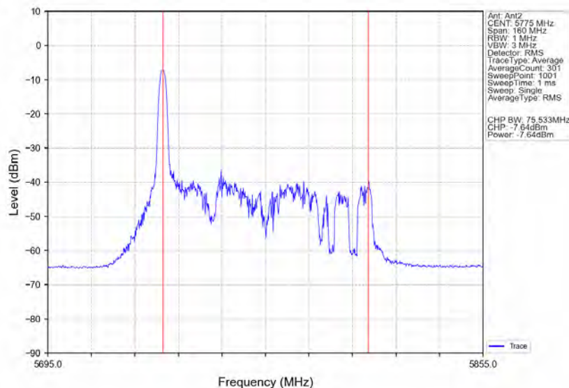
802.11ax(HE80) MCH_5775MHz RU26 Left Ant2 NTN
