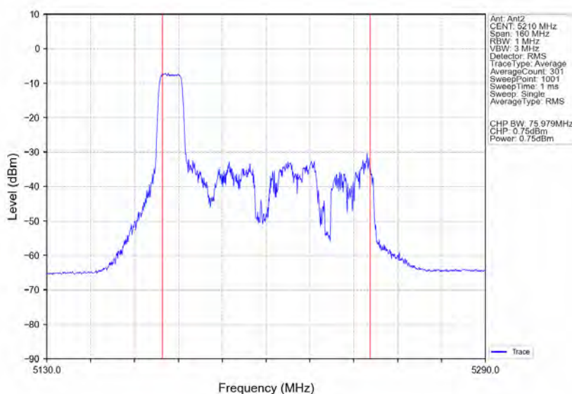
802.11ax(HE80) MCH 5210MHz RU106 Left Ant2 NTN
