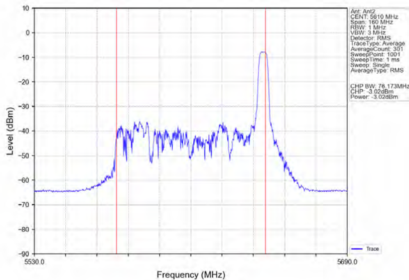
802.11ax(HE80) HCH 5610MHz RU52 Right Ant2 NTNv
