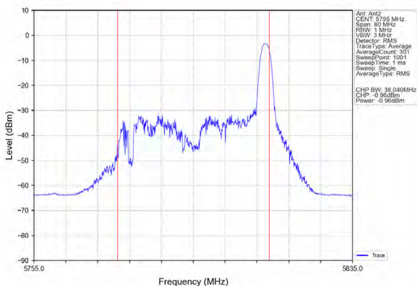
802.11ax(HE40) HCH 5795MHz RU26 Right Ant2 NTNv
