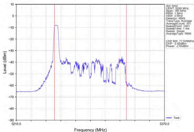
802.11ax(HE80) MCH_5290MHz RU52 Left Ant2 NTN
