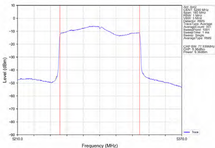
802.11ax(HE80) MCH 5290MHz RU996 Left Ant2 NTNv
