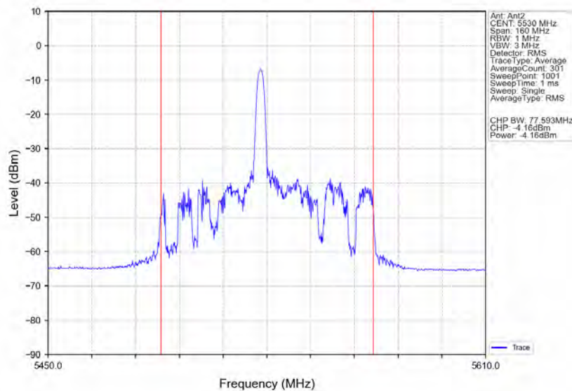
802.11ax(HE80) LCH 5530MHz RU26 Mid Ant2 NTNv
