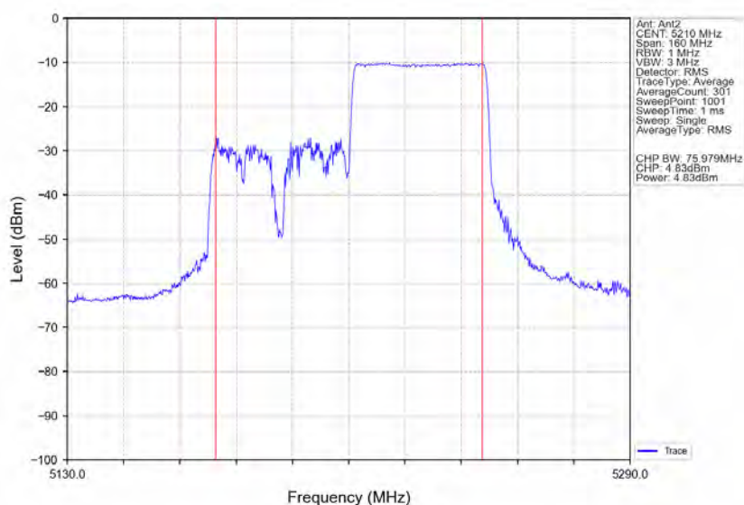
802.11ax(HE80) MCH 5210MHz RU484 Right Ant2 NTVN
