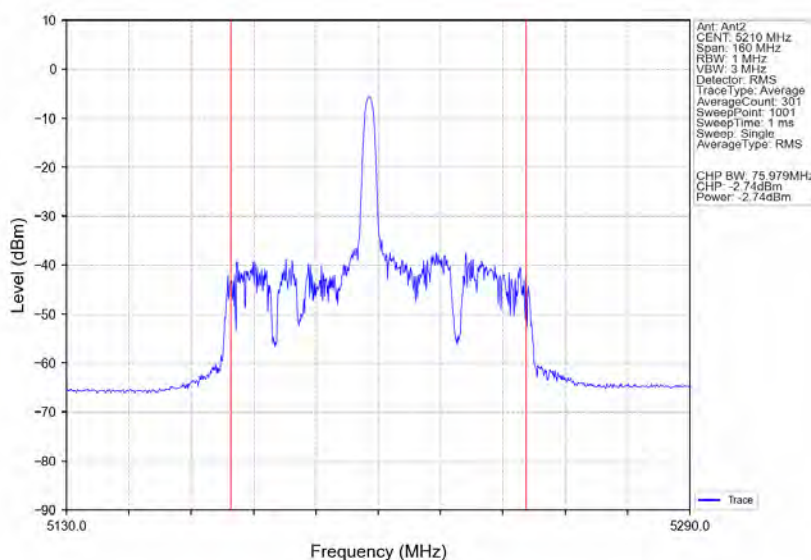
802.11ax(HE80) MCH_5210MHz RU26_Mid_Ant2_NTNV
