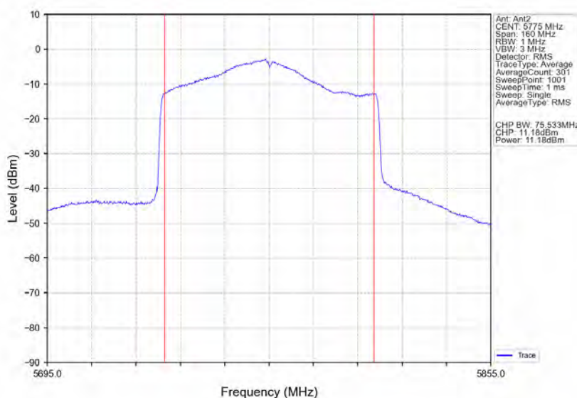
802.11ax(HE80) MCH 5775MHz RU996 Left Ant2 NTN
