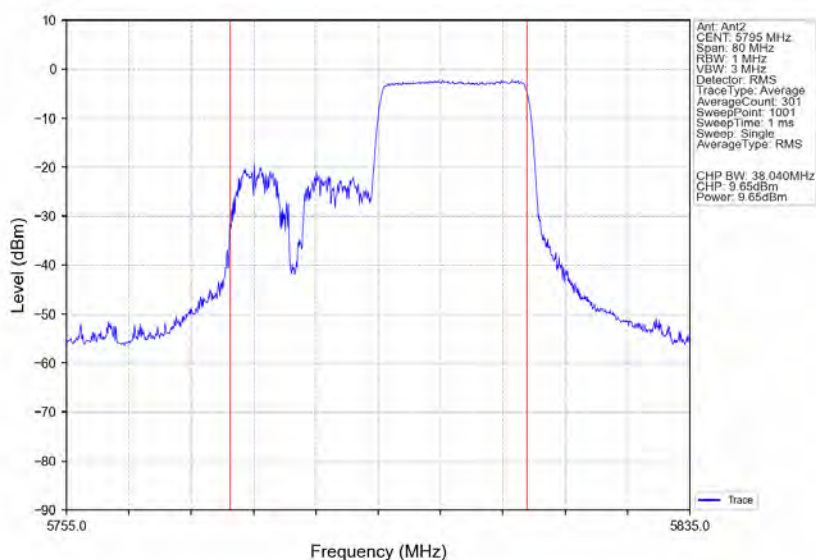
802.11ax(HE40) HCH 5795MHz RU242 Right Ant2 NTVN
