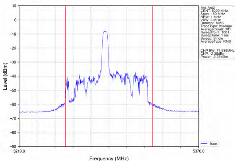
802.11ax(HE80) MCH_5290MHz RU52_Mid_Ant2_NTNV
