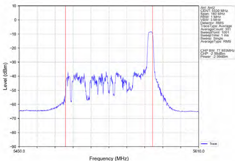
802.11ax(HE80) LCH 5530MHz RU52 Right Ant2 NTNv
