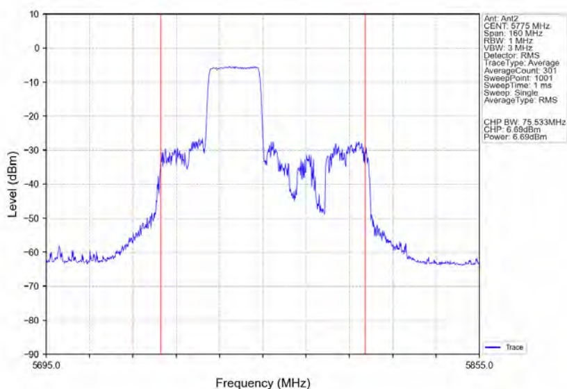
802.11ax(HE80) MCH 5775MHz RU242 Mid Ant2 NTNv
