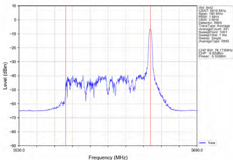
802.11ax(HE80) HCH 5610MHz RU26 Right Ant2 NTNv
