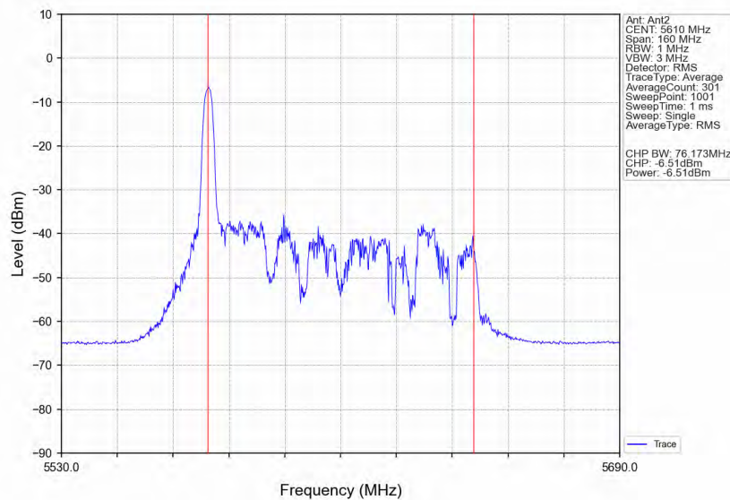
802.11ax(HE80) HCH 5610MHz RU26 Left Ant2 NTN
