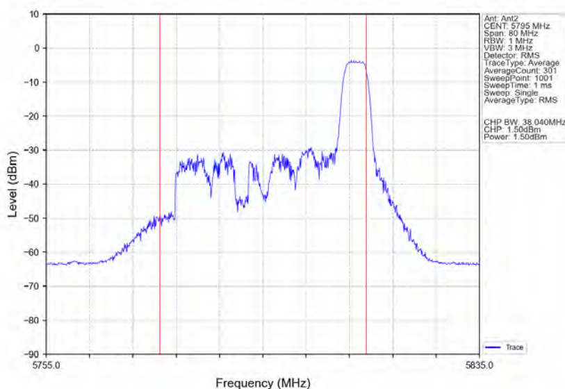
802.11ax(HE40) HCH 5795MHz RU52 Right Ant2 NTNv
