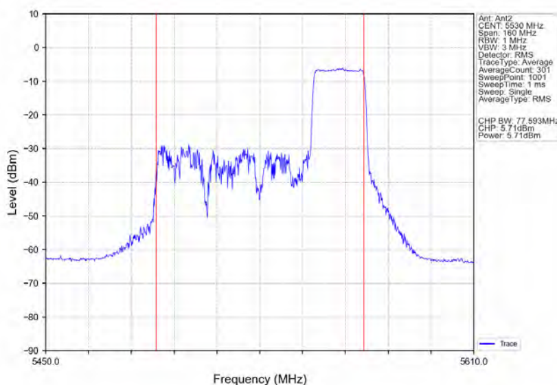
802.11ax(HE80) LCH 5530MHz RU242 Right Ant2 NTVN
