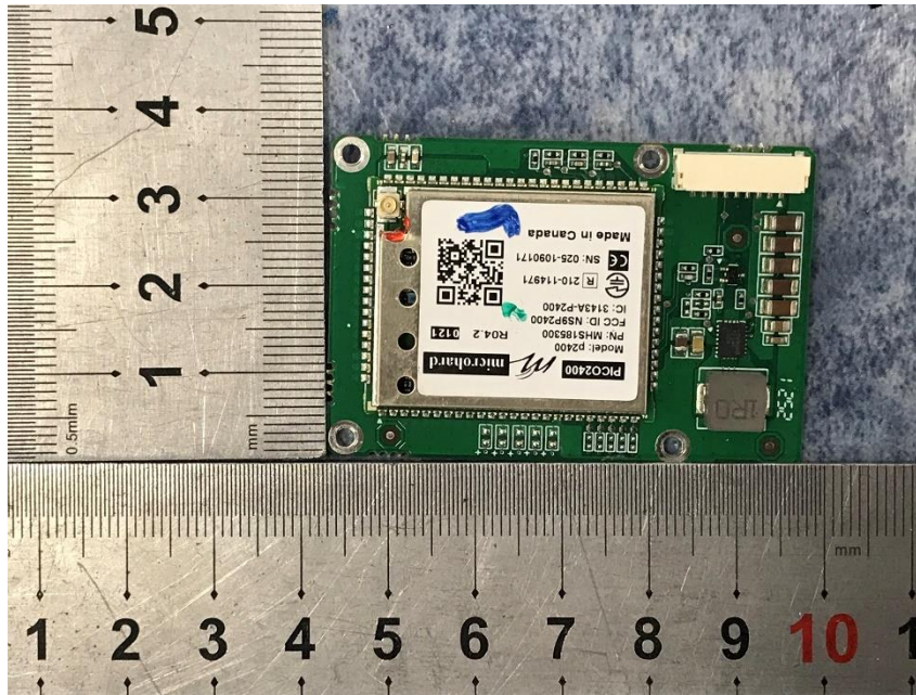
2.4G module p2400(FCC ID: NS9P2400)
