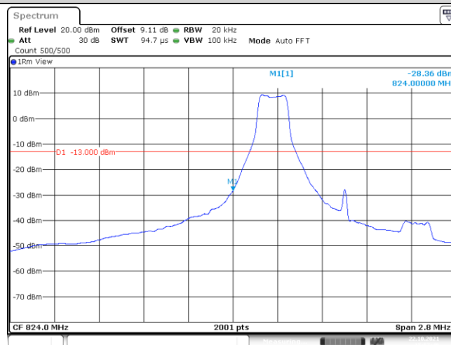
Band5-1.4MHz-QPSK-20407-1-0-Low--28.36-PASS
