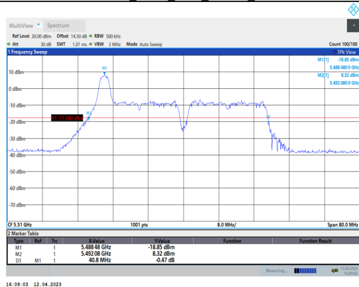
11AX40_Ant10_5510_52Tone_RU37
