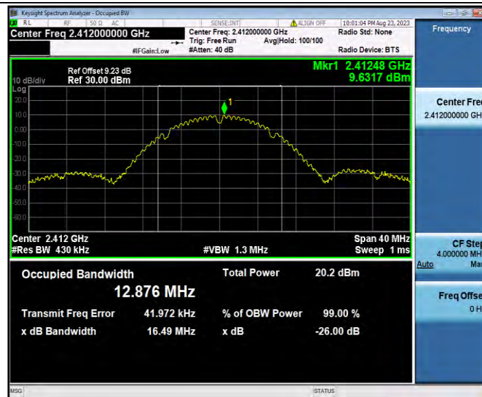
11B_Ant0_2412
