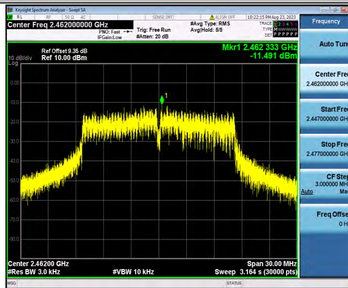
11G_Ant0_2462
