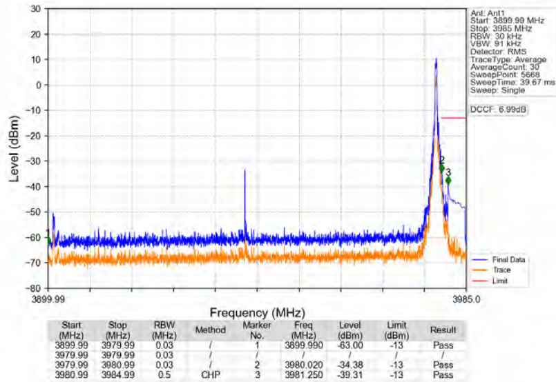
n77a 30kHz SISO NTN 80MHz CP-OFDM QPSK 3939.99MHz Edge 1RB Right
