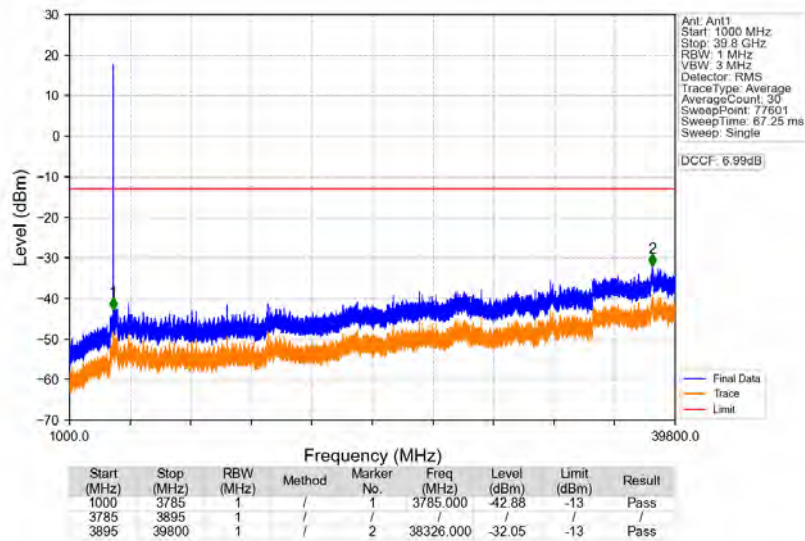
n77a 30kHz SISO NTN 100MHz CP-OFDM QPSK 3840MHz Edge 1RB Left
