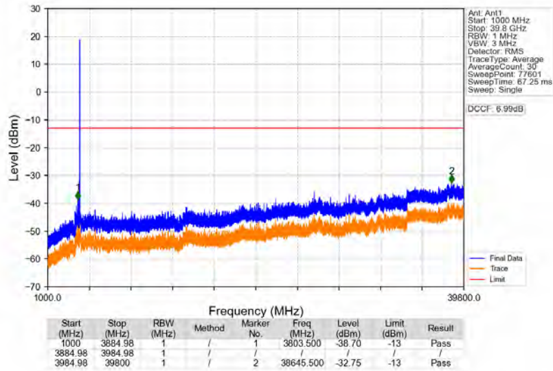
n77a 30kHz SISO NTN 90MHz CP-OFDM QPSK 3934.98MHz Edge 1RB Right
