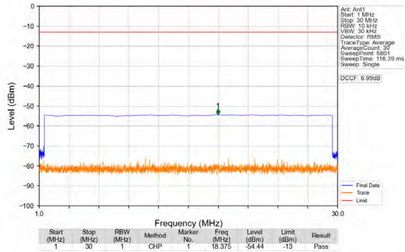
n77a 30kHz SISO NTN 80MHz CP-OFDM QPSK 3939.99MHz Edge 1RB Right
