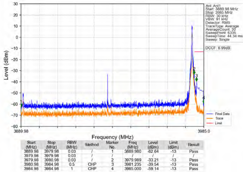
n77a 30kHz SISO NTN 90MHz CP-OFDM QPSK 3934.98MHz Edge 1RB Right
