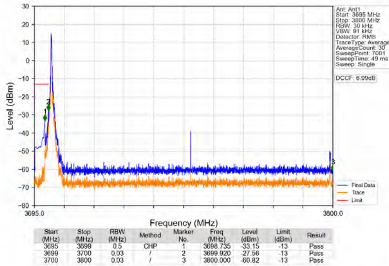
n77a 30kHz SISO NTN 100MHz DFT-s-OFDM QPSK 3750MHz Edge 1RB Left
