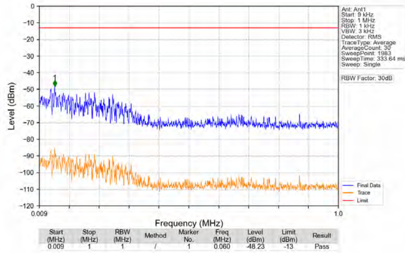
n77a 30kHz SISO NTN 100MHz CP-OFDM QPSK 3840MHz Edge 1RB Left
