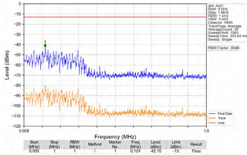
n77a 30kHz SISO NTN 100MHz DFT-s-OFDM QPSK 3840MHz Edge 1RB Left
