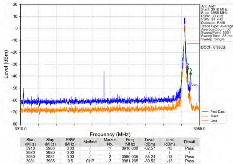
n77a 30kHz SISO NTN 70MHz CP-OFDM QPSK 3945MHz Edge 1RB Right
