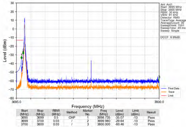
n77a 30kHz SISO NTN 100MHz CP-OFDM QPSK 3750MHz Edge 1RB Left
