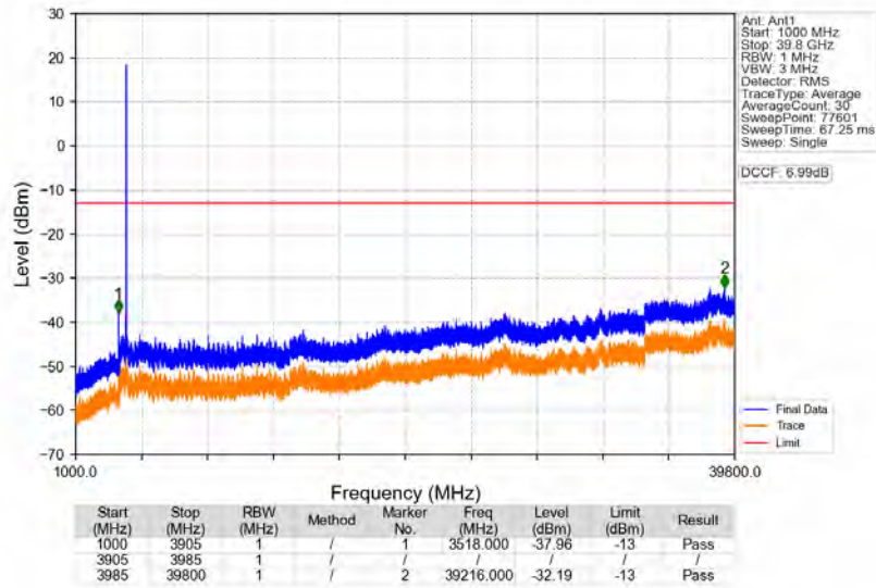
n77a 30kHz SISO NTN 70MHz DFT-s-OFDM QPSK 3945MHz Edge 1RB_Right
