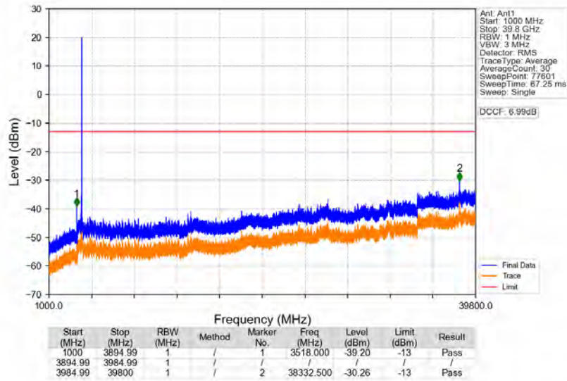
n77a 30kHz SISO NTN 80MHz CP-OFDM QPSK 3939.99MHz Edge 1RB Right
