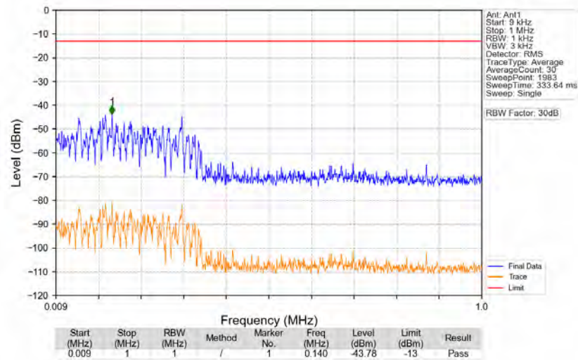
n77a 30kHz SISO NTN 100MHz DFT-s-OFDM QPSK 3750MHz Edge 1RB Left
