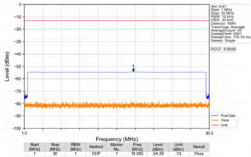
n77a 30kHz SISO NTN 100MHz CP-OFDM QPSK 3750MHz Edge 1RB Left
