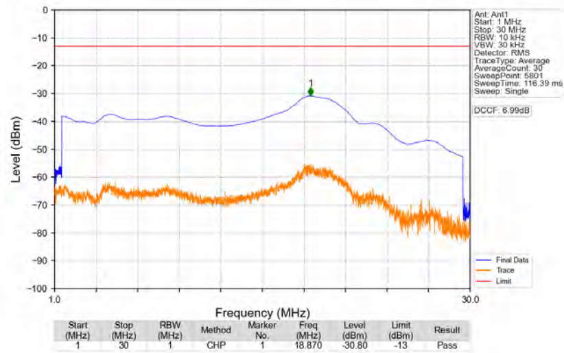
n77a 30kHz SISO NTN 90MHz CP-OFDM QPSK 3934.98MHz Edge 1RB Right
