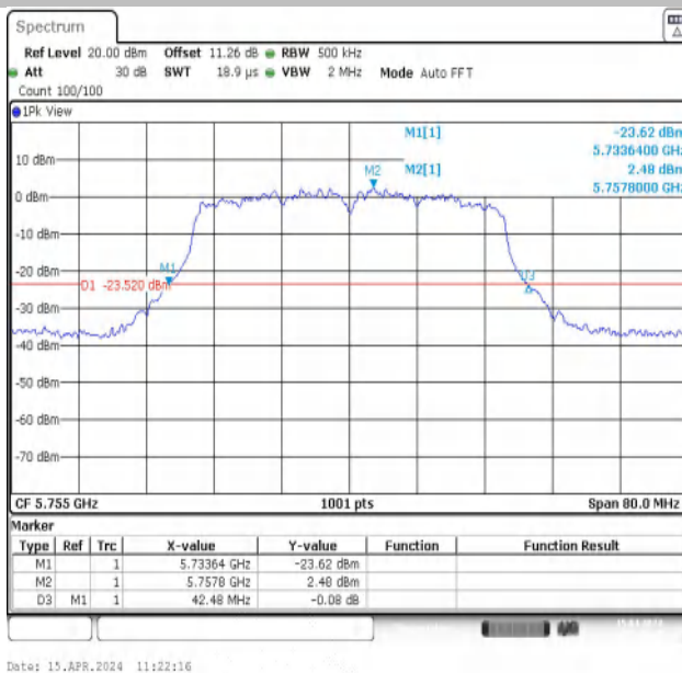
11N40MIMO-Ant1-5755
