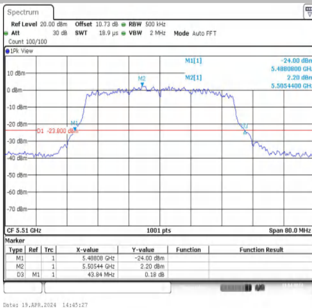
11AX40MIMO-Ant1-5510
