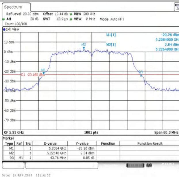
11N40MIMO-Ant1-5230
