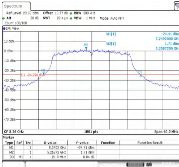
11AC20MIMO-Ant1-5260
