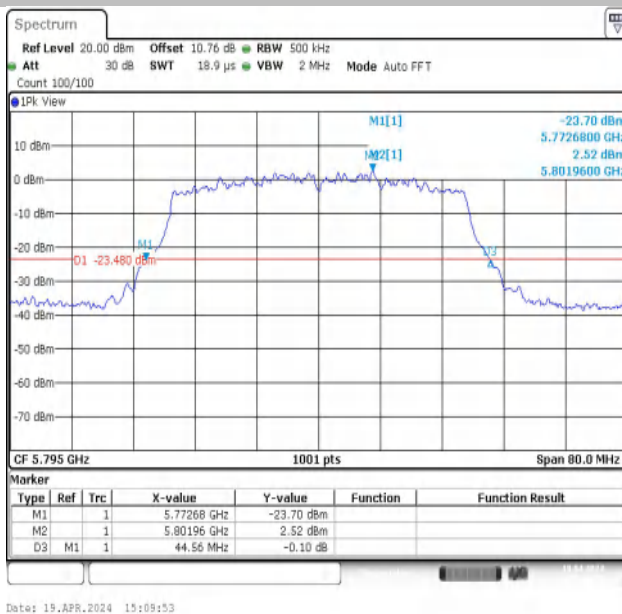
11AX40MIMO-Ant1-5795
