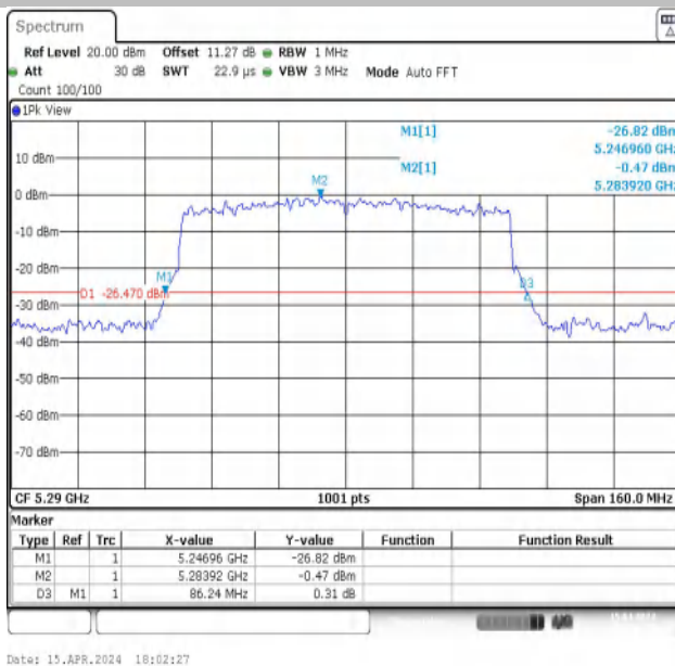
11AX80MIMO-Ant1-5290
