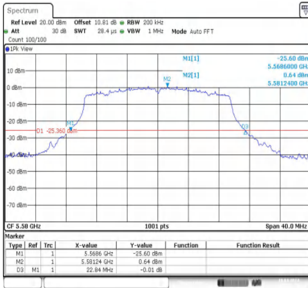
11AX20MIMO-Ant1-5580
