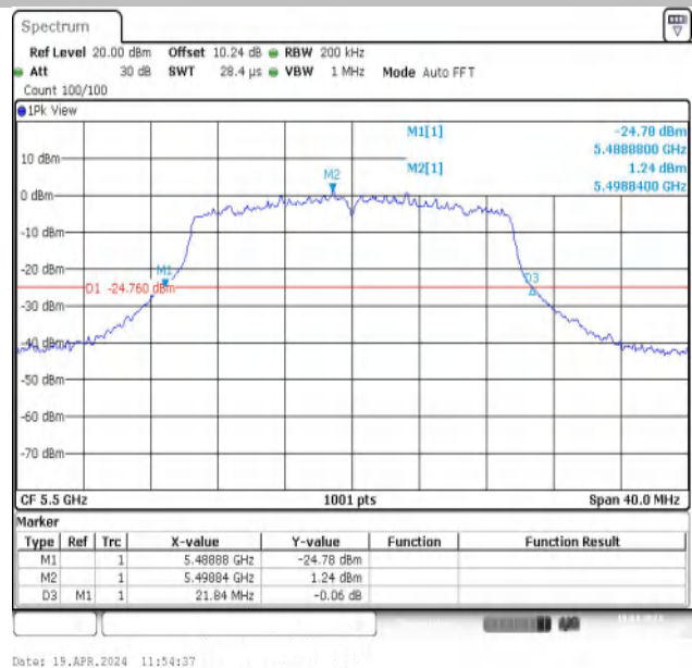
11AX20MIMO-Ant2-5500
