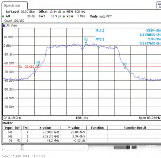
11N40MIMO-Ant1-5190
