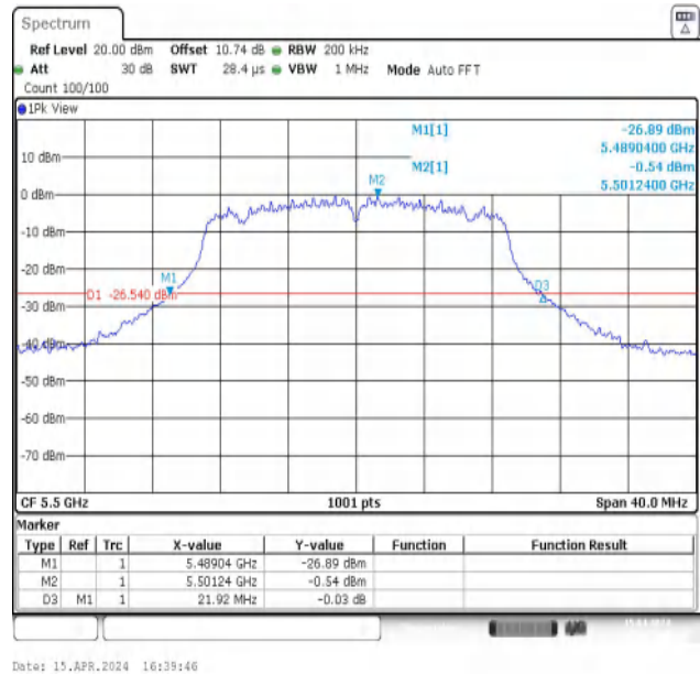
11N20MIMO-Ant2-5500
