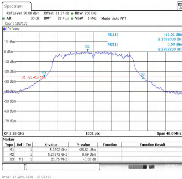
11N20MIMO-Ant1-5280
