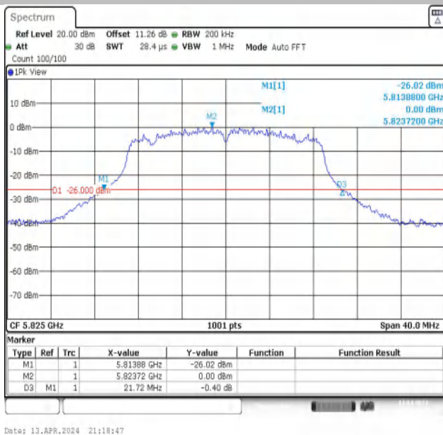
11N20MIMO-Ant1-5825
