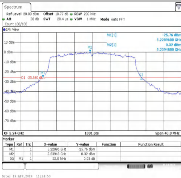
11AX20MIMO-Ant1-5240
