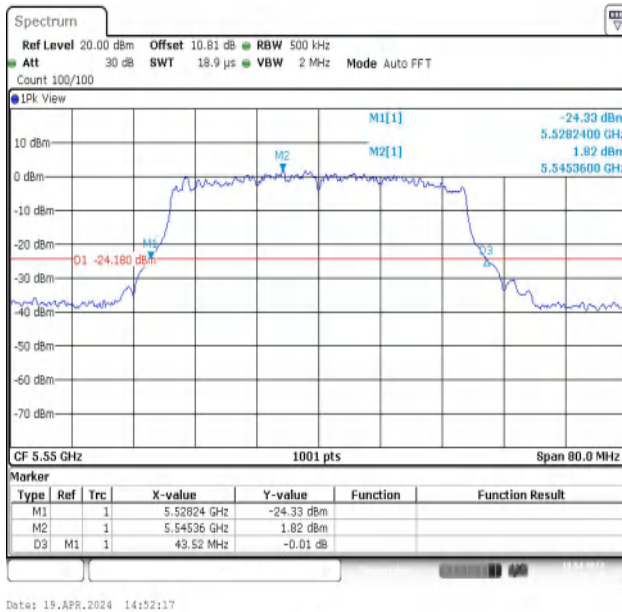
11AX40MIMO-Ant1-5550
