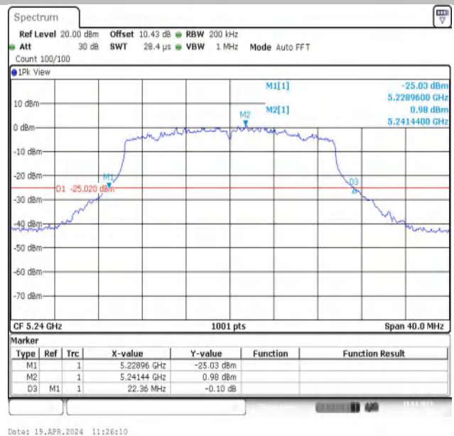
11AX20MIMO-Ant2-5240
