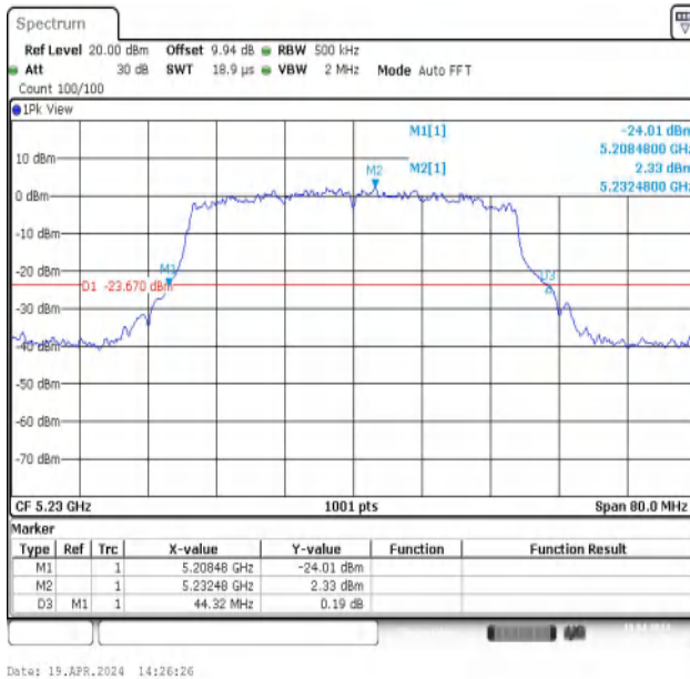
11AX40MIMO-Ant1-5230
