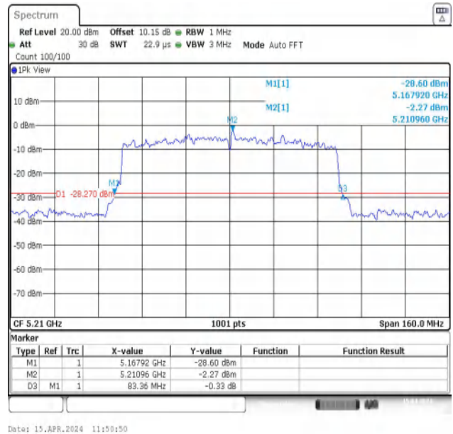
11AX80MIMO-Ant2-5210
