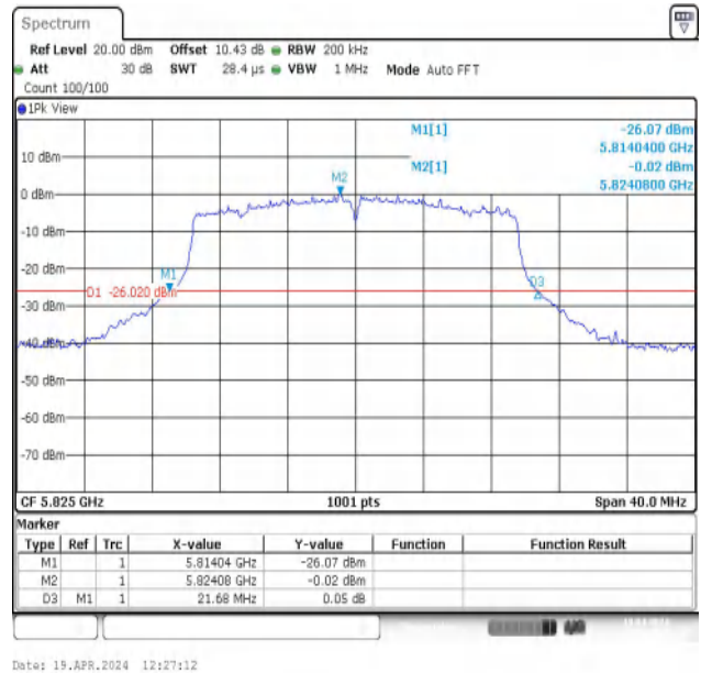
11AX20MIMO-Ant2-5825
