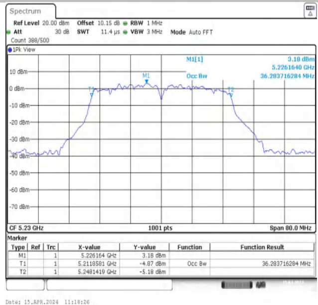
11N40MIMO-Ant2-5230
