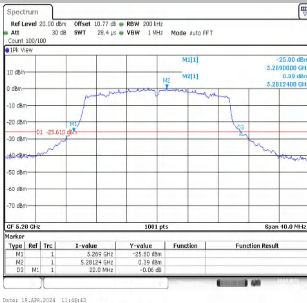
11AX20MIMO-Ant1-5280
