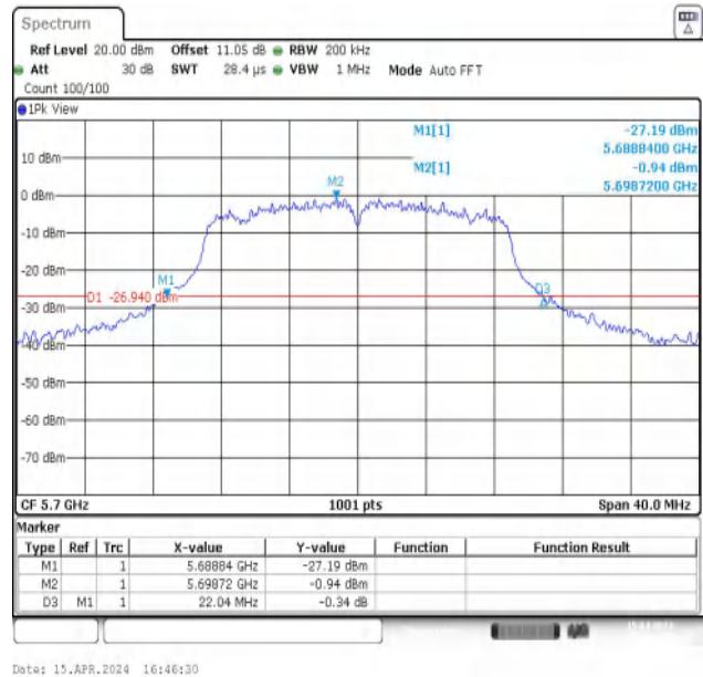
11N20MIMO-Ant2-5700
