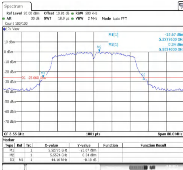
11AC40MIMO-Ant1-5550
