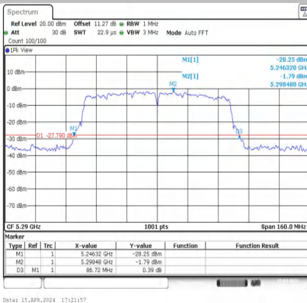
11AC80MIMO-Ant1-5290
