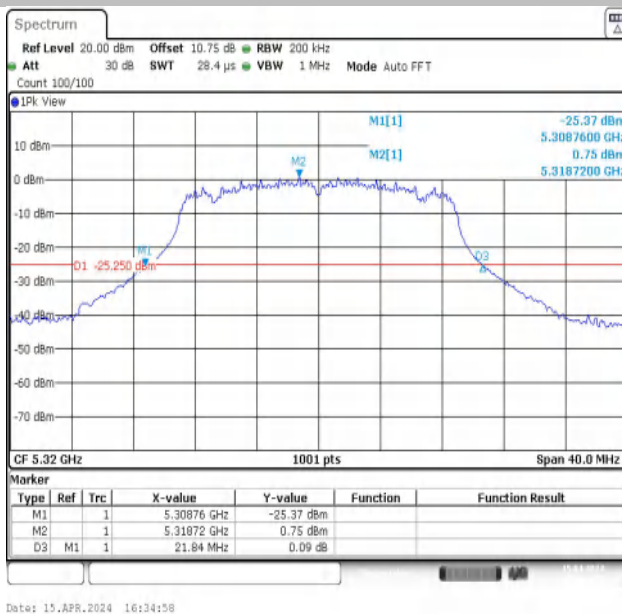
11N20MIMO-Ant1-5320
