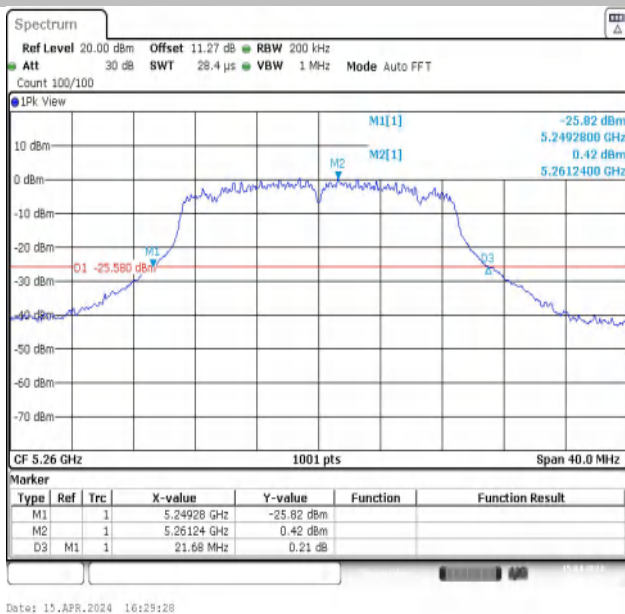
11N20MIMO-Ant1-5260
