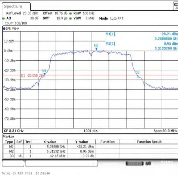
11N40MIMO-Ant1-5310
