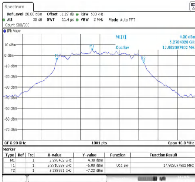
11N20MIMO-Ant1-5280
