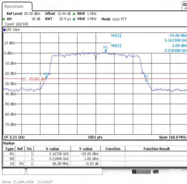
11AC80MIMO-Ant1-5210
