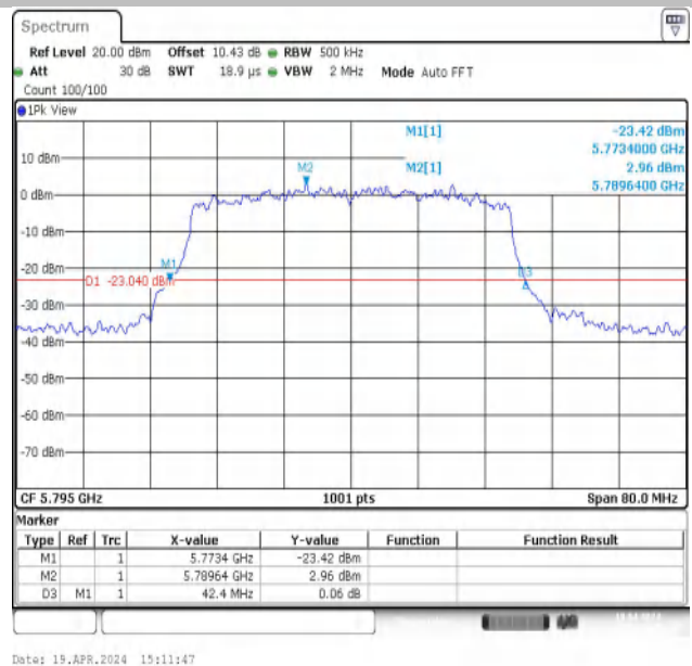
11AX40MIMO-Ant2-5795
