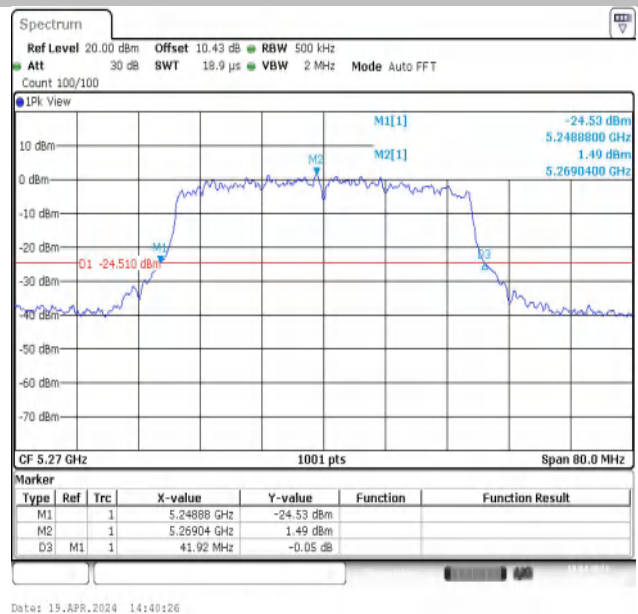
11AX40MIMO-Ant2-5270
