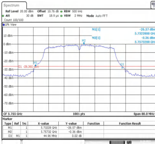
11AC40MIMO-Ant1-5755
