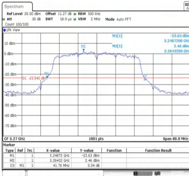
11N40MIMO-Ant1-5270
