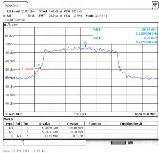
11AX40MIMO-Ant2-5230
