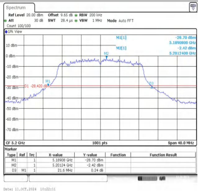
11N20MIMO-Ant2-5200
