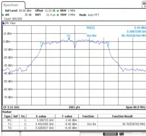
11N40MIMO-Ant1-5510
