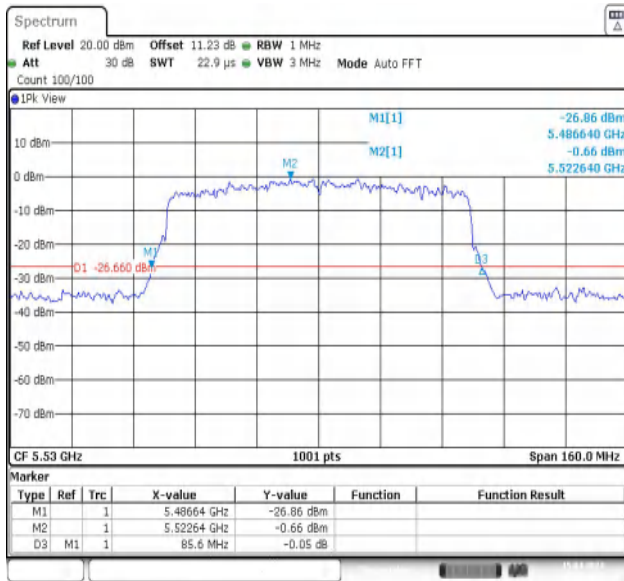
11AX80MIMO-Ant1-5530
