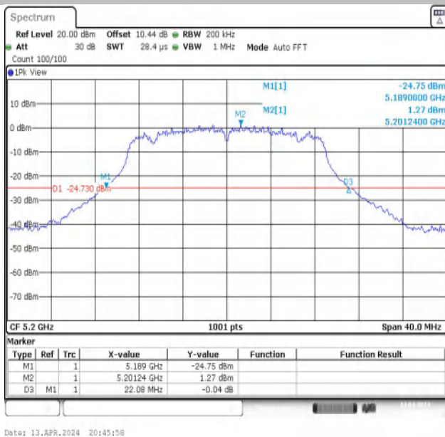
11N20MIMO-Ant1-5200
