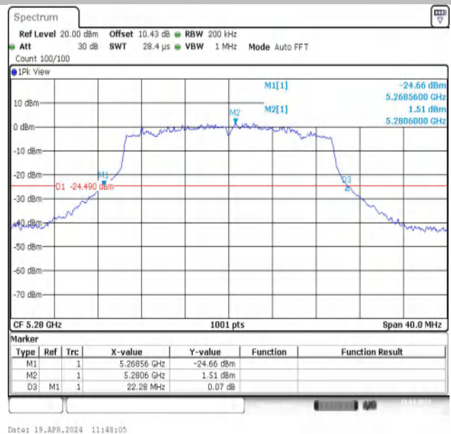
11AX20MIMO-Ant2-5280
