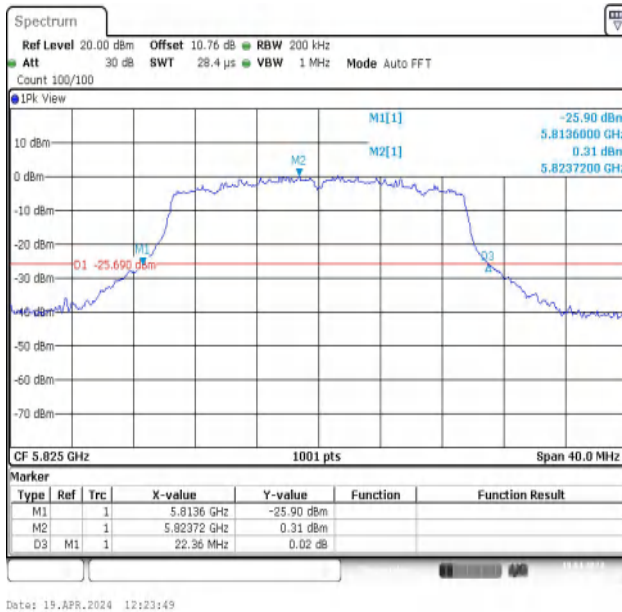
11AX20MIMO-Ant1-5825
