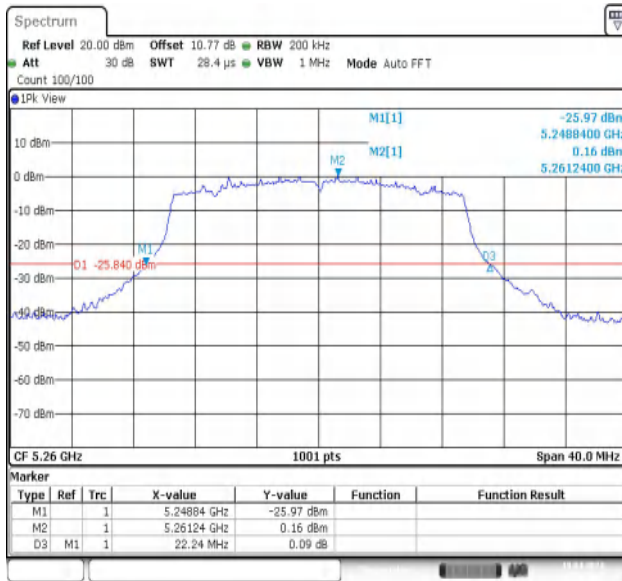
11AX20MIMO-Ant1-5260
