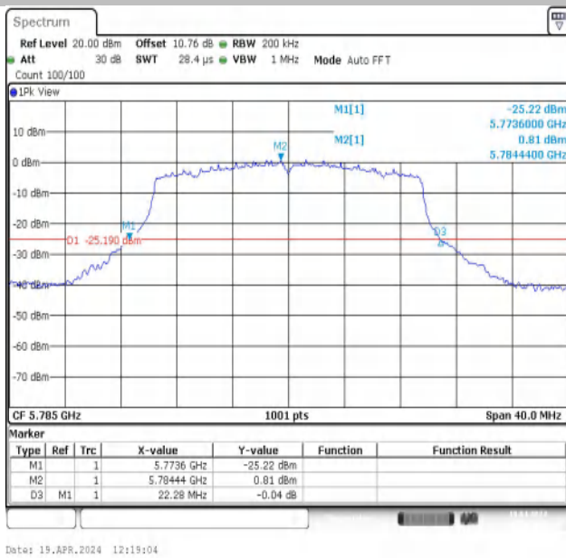
11AX20MIMO-Ant1-5785
