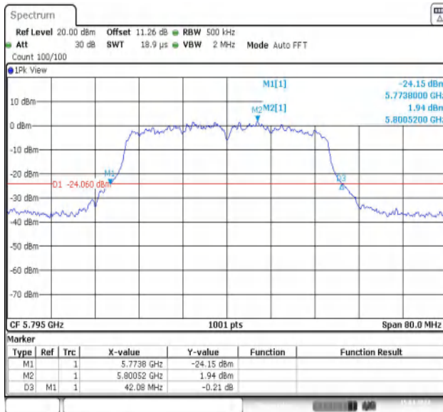
11N40MIMO-Ant1-5795
