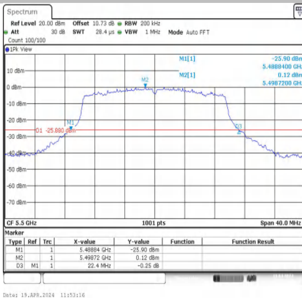
11AX20MIMO-Ant1-5500
