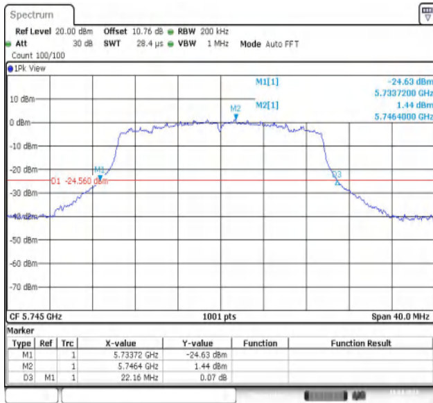
11AX20MIMO-Ant1-5745
