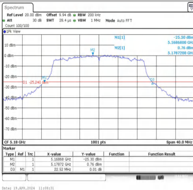
11AX20MIMO-Ant1-5180
