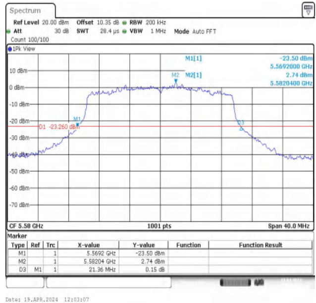
11AX20MIMO-Ant2-5580
