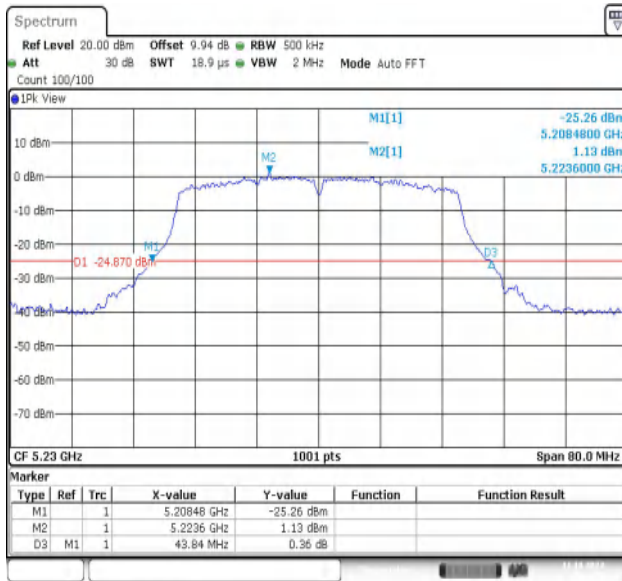
11AC40MIMO-Ant1-5230
