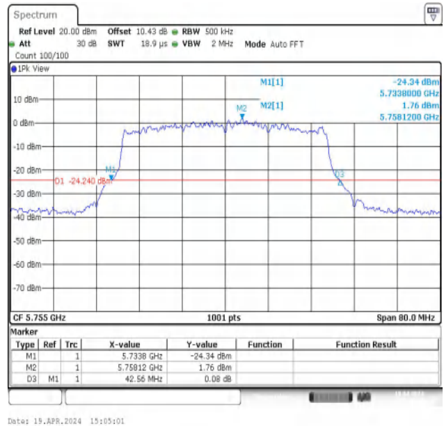
11AX40MIMO-Ant2-5755
