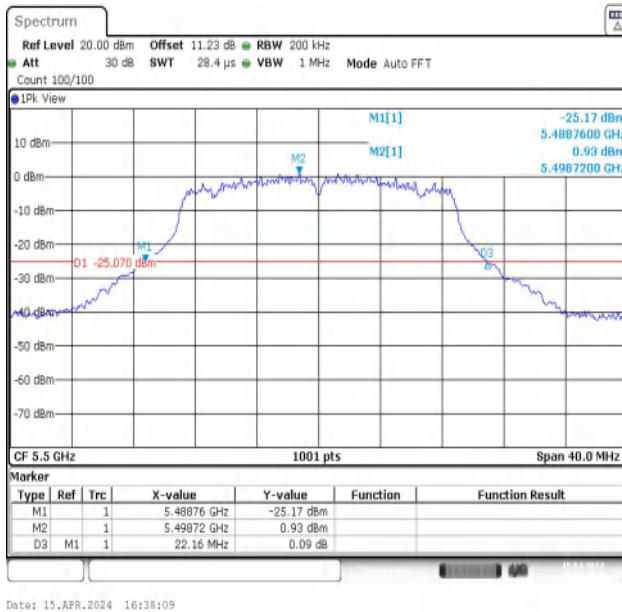
11N20MIMO-Ant1-5500
