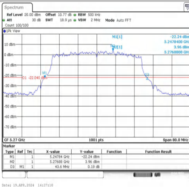
11AX40MIMO-Ant1-5270
