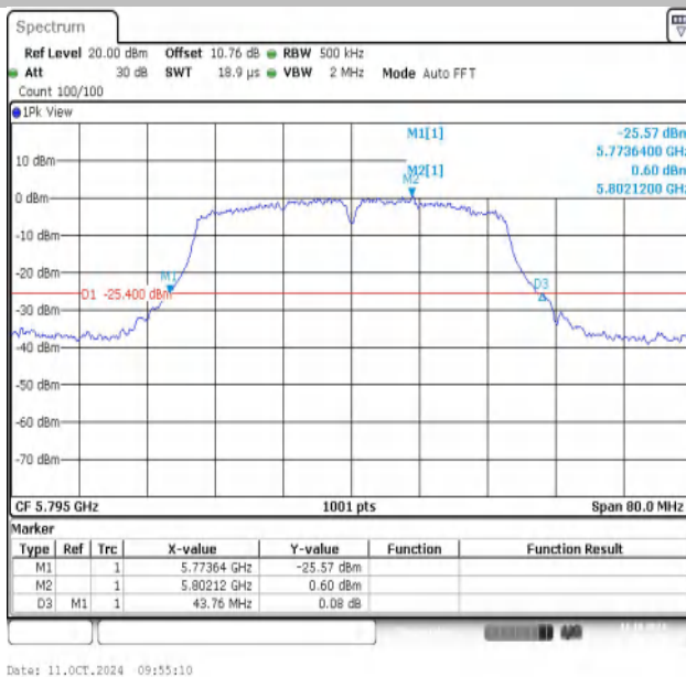
11AC40MIMO-Ant1-5795
