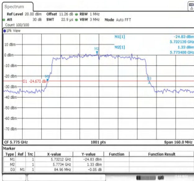
11AX80MIMO-Ant1-5775
