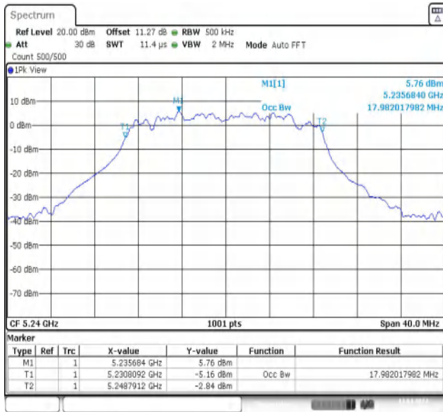
11N20MIMO-Ant1-5240
