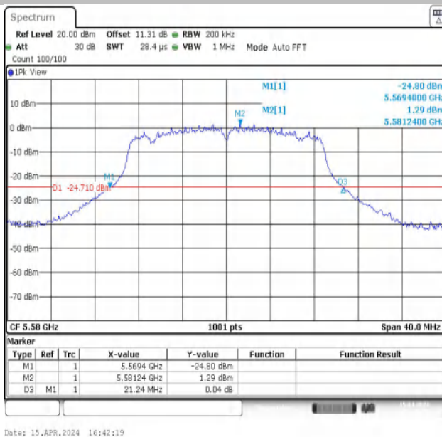
11N20MIMO-Ant1-5580
