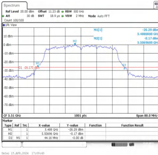
11N40MIMO-Ant1-5510
