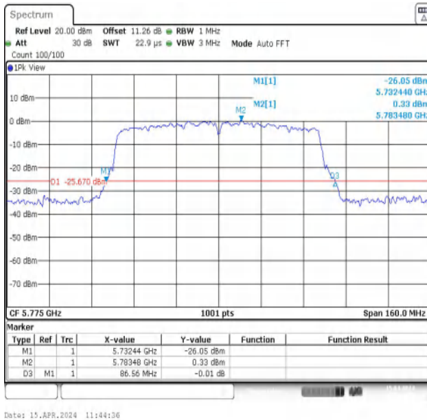
11AC80MIMO-Ant1-5775
