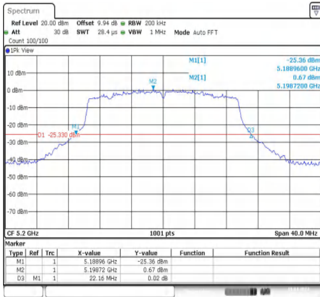
11AX20MIMO-Ant1-5200
