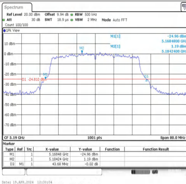
11AX40MIMO-Ant1-5190
