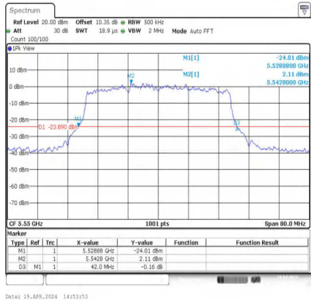
11AX40MIMO-Ant2-5550
