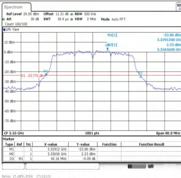
11N40MIMO-Ant1-5550
