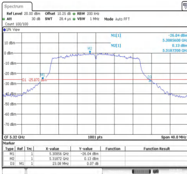
11AX20MIMO-Ant1-5320
