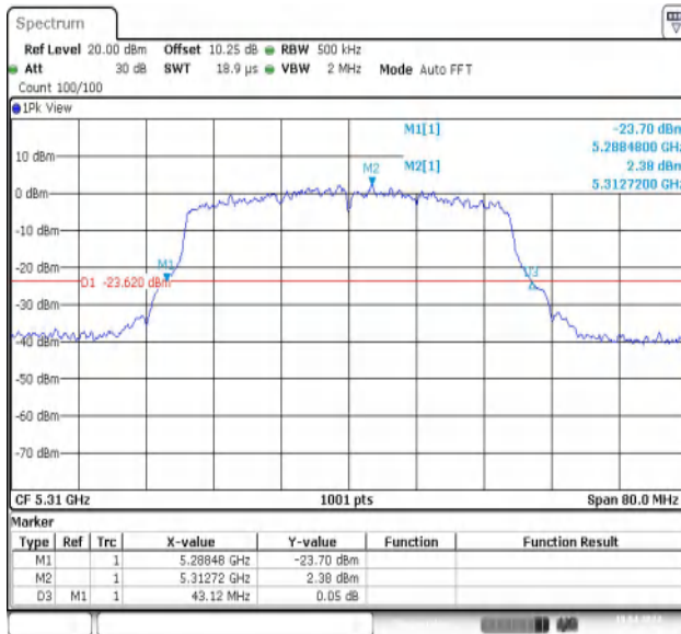
11AX40MIMO-Ant1-5310
