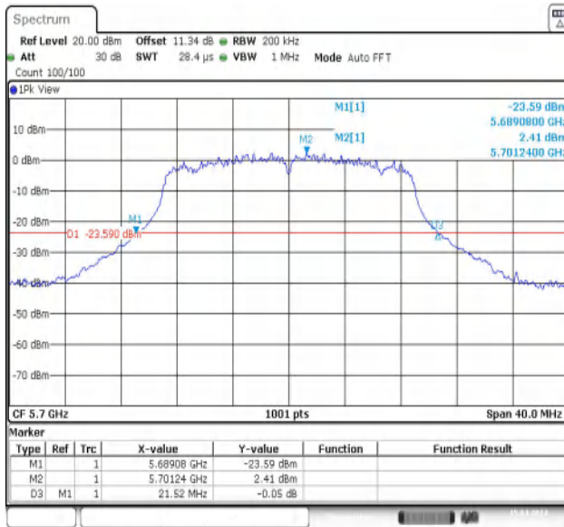
11N20MIMO-Ant1-5700
