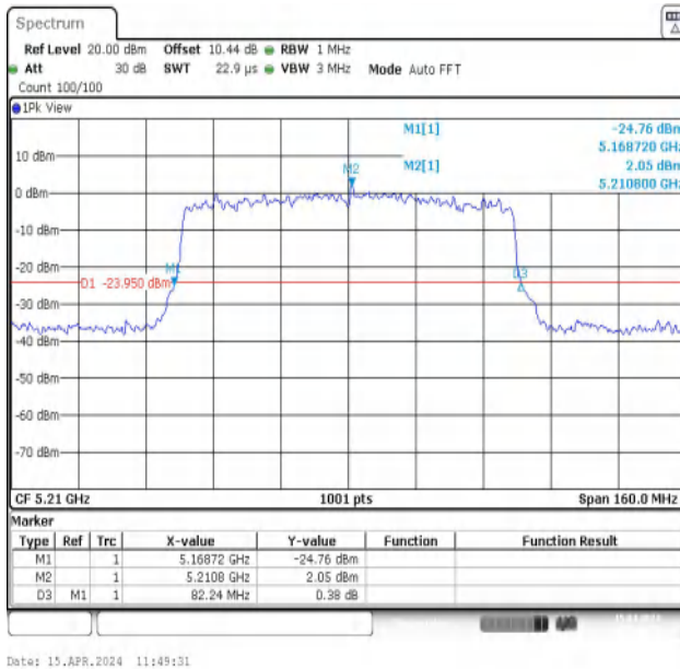
11AX80MIMO-Ant1-5210
