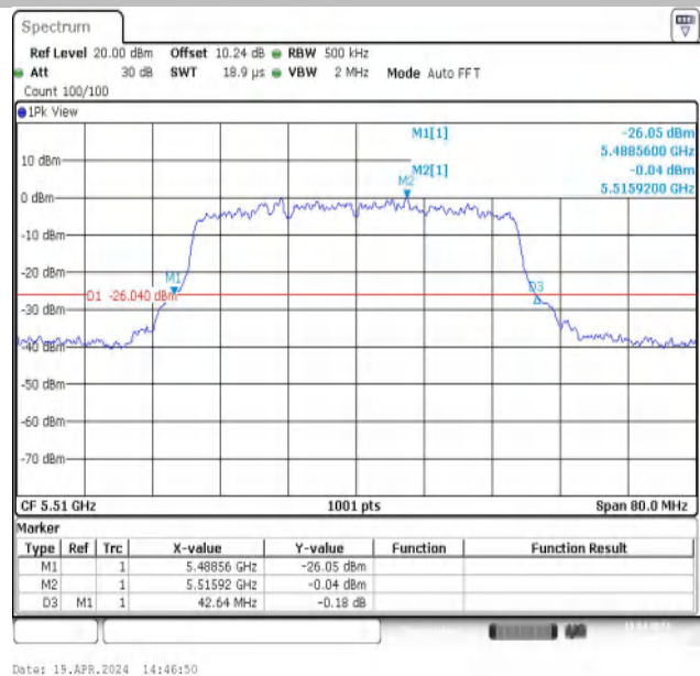
11AX40MIMO-Ant2-5510
