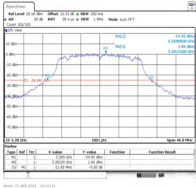
11N20MIMO-Ant2-5280
