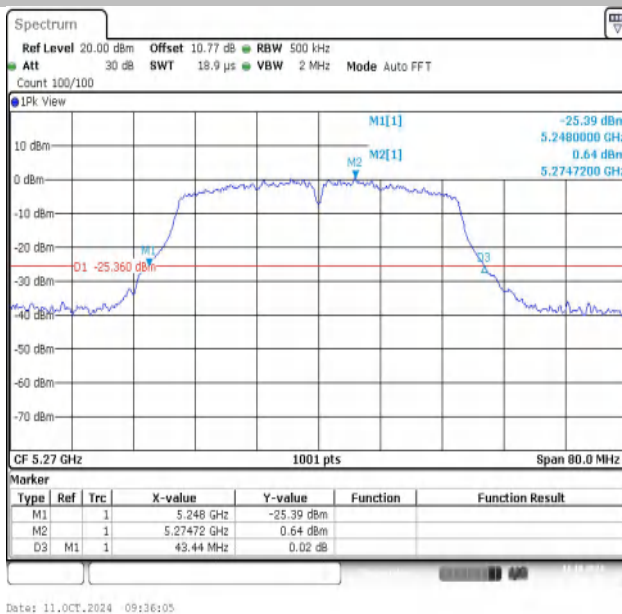
11AC40MIMO-Ant1-5270
