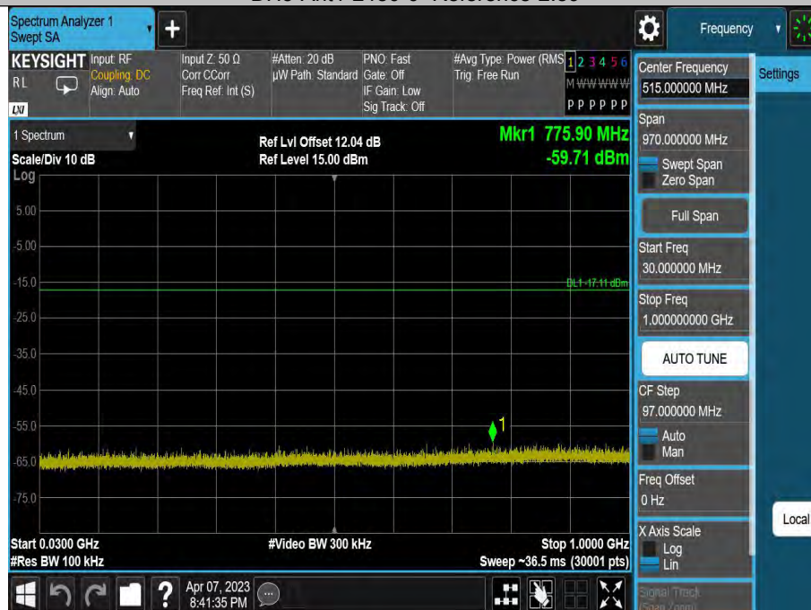
DH5-Ant1-2480-30~1000-2.89
