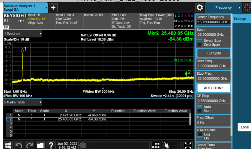
11N40_Ant1_2437_0~Reference
