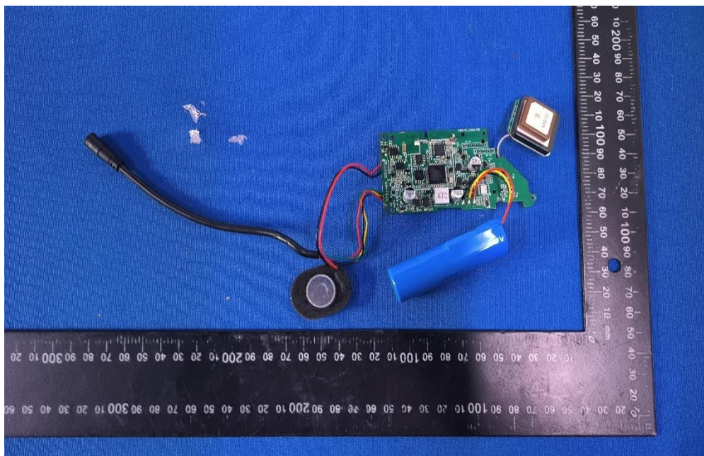
(6) EUT Photo
