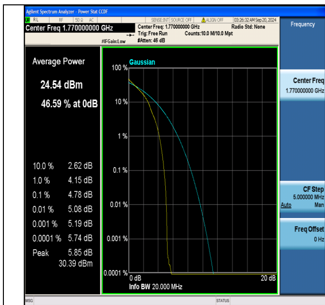
Band66-20MHz-QPSK-132572-1RB#0-PASS
