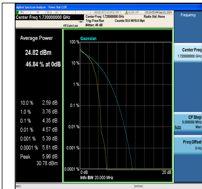
Band66-20MHz-QPSK-132072-1RB#0-PASS
