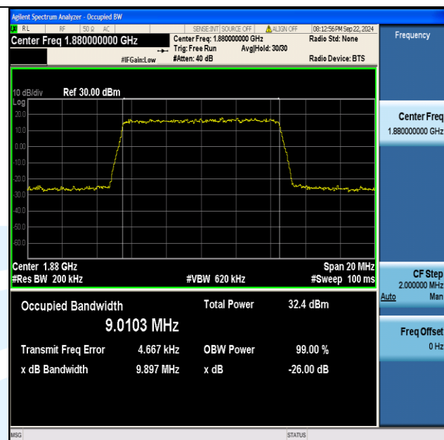
Band2-10MHz-QPSK-18900-50RB#0-PASS
