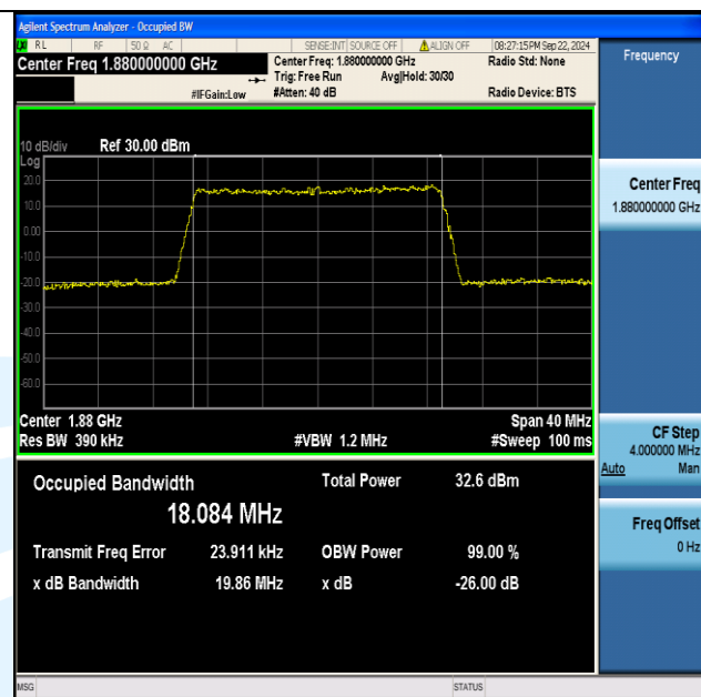
Band2-20MHz-QPSK-18900-100RB#0-PASS
