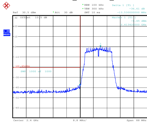
802.11n20_2412MHz_Chain 2
