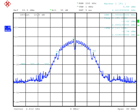
802.11b_2412MHz_Chain 2
