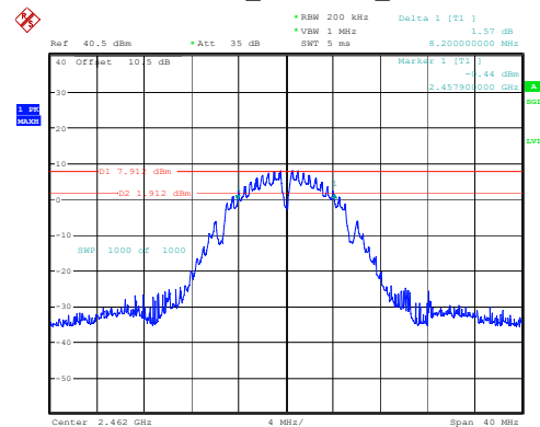
802.11b_2462MHz_Chain 2
