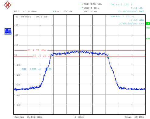
802.11n20_2412MHz_Chain 2
