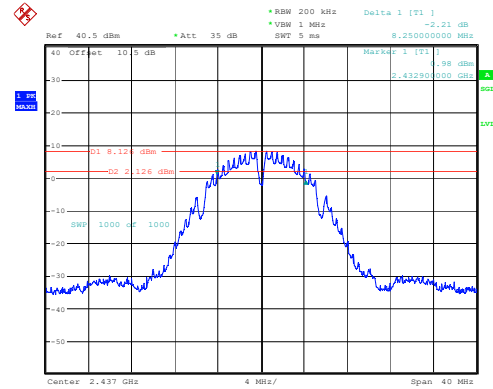
802.11b_2437MHz_Chain 1
