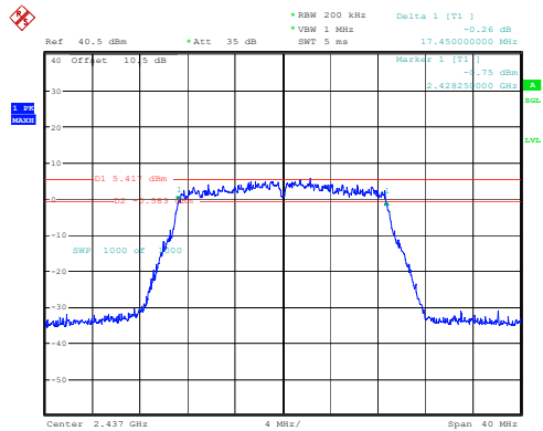
802.11n20_2437MHz_Chain 2
