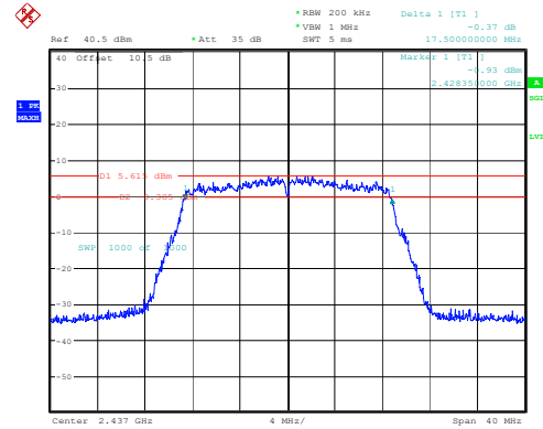
802.11n20_2437MHz_Chain 1
