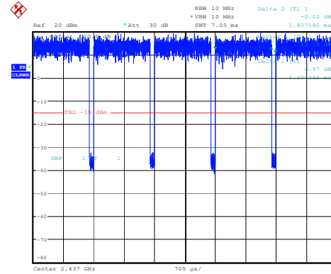
802.11n20_2437MHz_Chain 2
