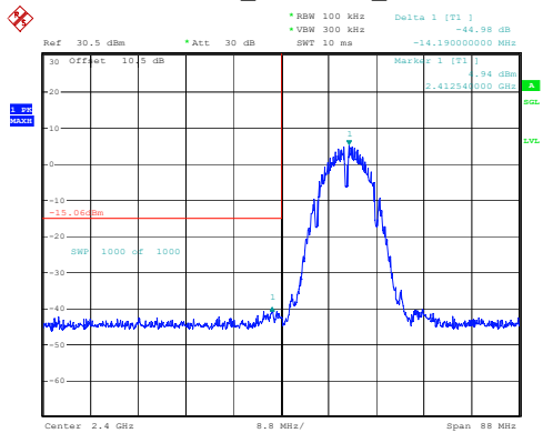
802.11b_2412MHz_Chain 1
