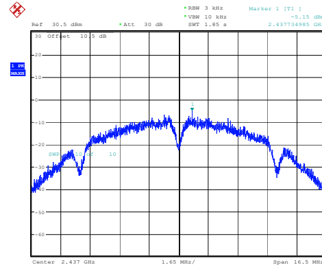
802.11b_2437MHz_Chain 1
