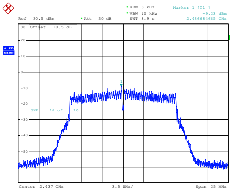
802.11n20_2437MHz_Chain 1
