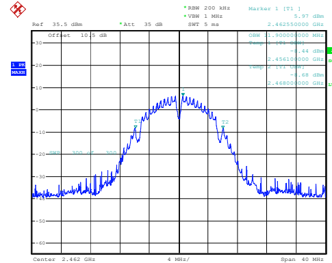
802.11b_2462MHz_Chain 2
