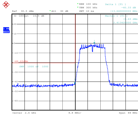
802.11n20_2412MHz_Chain 1
