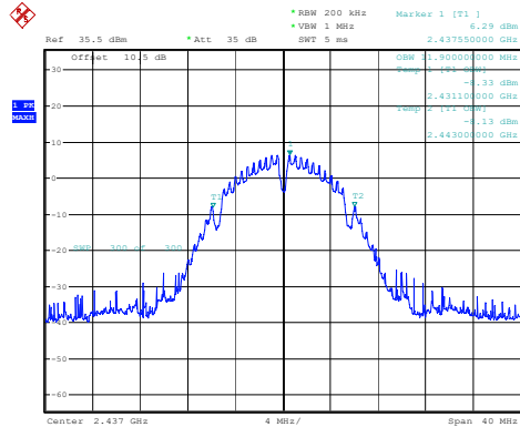
802.11b_2437MHz_Chain 2
