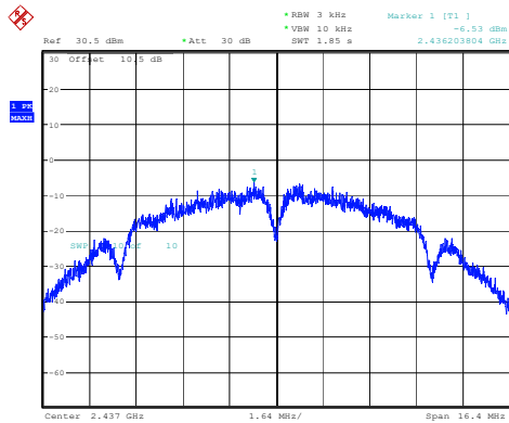
802.11b_2437MHz_Chain 2
