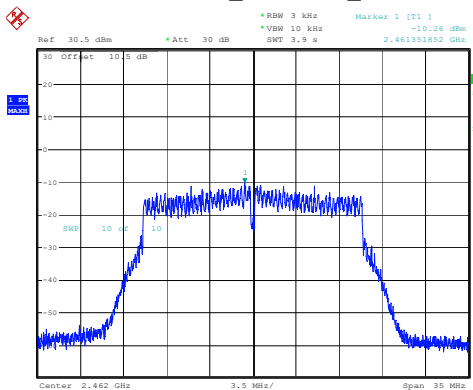
802.11n20_2462MHz_Chain 2
