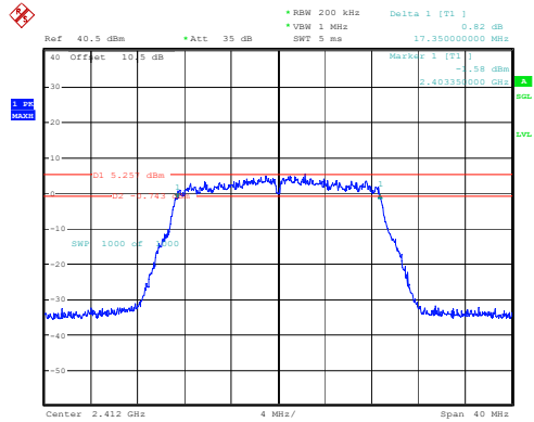
802.11n20_2412MHz_Chain 1
