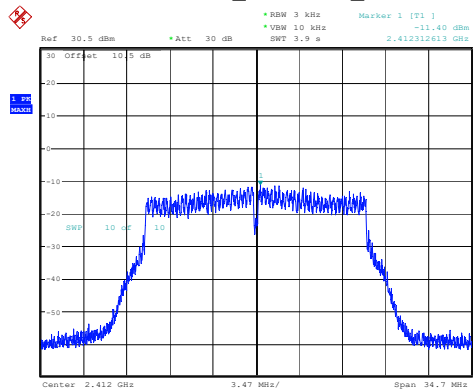
802.11n20_2412MHz_Chain 1
