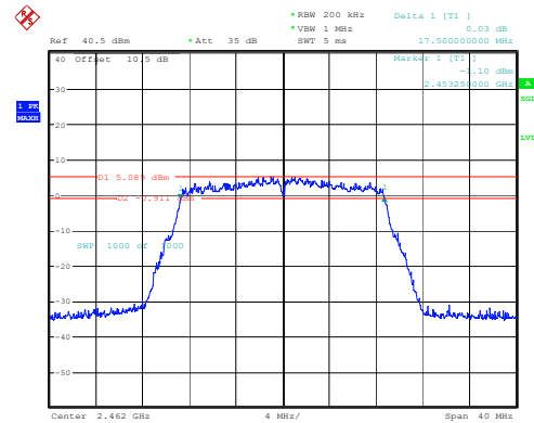
802.11n20_2462MHz_Chain 2
