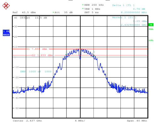
802.11b_2437MHz_Chain 2
