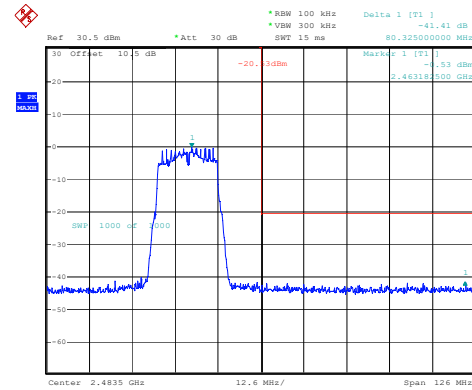
802.11n20_2462MHz_Chain 1
