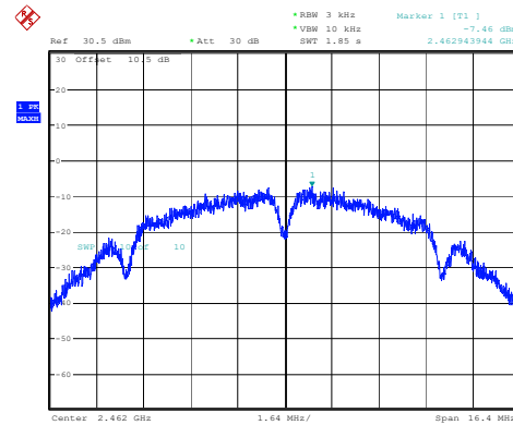
802.11b_2462MHz_Chain 2
