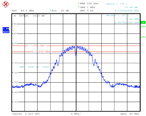
802.11b_2412MHz_Chain 1
