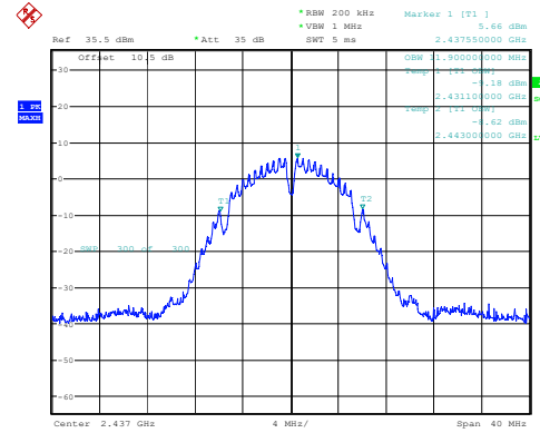
802.11b_2437MHz_Chain 1
