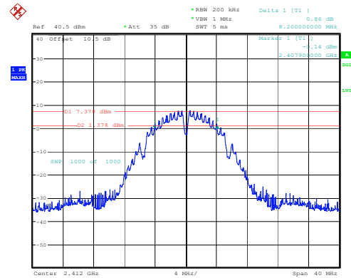
802.11b_2412MHz_Chain 2
