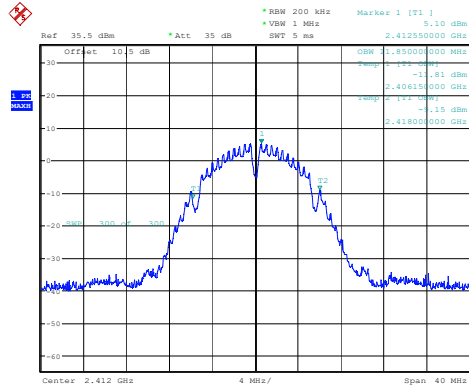
802.11b_2412MHz_Chain 1
