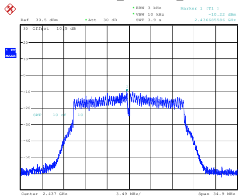
802.11n20_2437MHz_Chain 2
