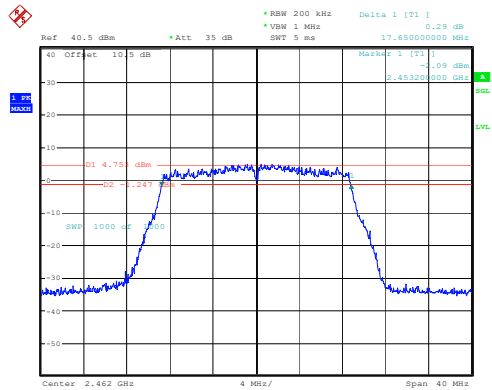
802.11n20_2462MHz_Chain 1
