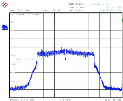
802.11n20_2412MHz_Chain 2
