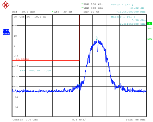
802.11b_2412MHz_Chain 2
