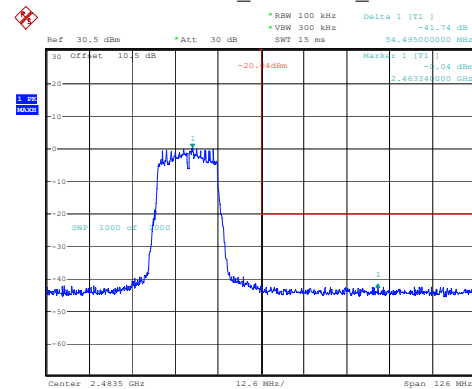
802.11n20_2462MHz_Chain 2
