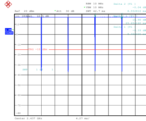
802.11b_2437MHz_Chain 2
