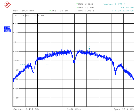
802.11b_2412MHz_Chain 2
