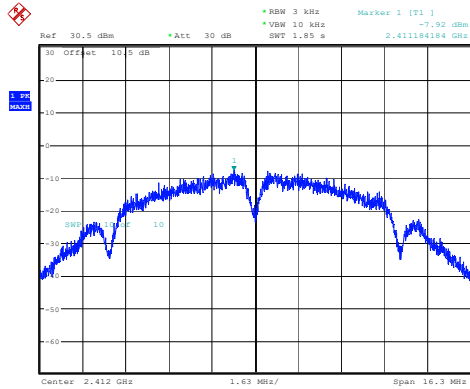
802.11b_2412MHz_Chain 1
