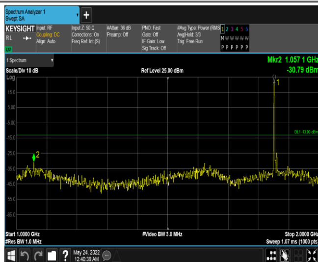
Band25-5MHz-QPSK-26065-1RB#0-Range2:1000~2000MHz
