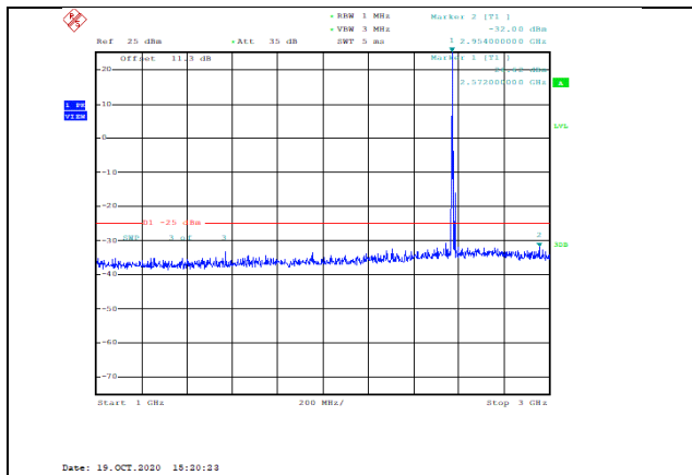
Band38-5MHz-QPSK-37775-1RB#0-Range2:1000~3000MHz--32-PASS
