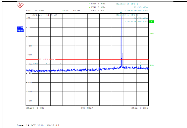
Band7-20MHz-QPSK-21350-1RB#0-Range2:1000~3000MHz--31.93-PASS
