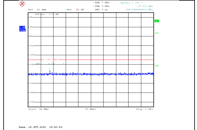
Band41-5MHz-QPSK-40065-1RB#0-Range1:30~1000MHz--37.83-PASS
