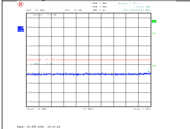
Band41-20MHz-QPSK-40590-1RB#0- Range1:30~1000MHz--38.05-PASS
