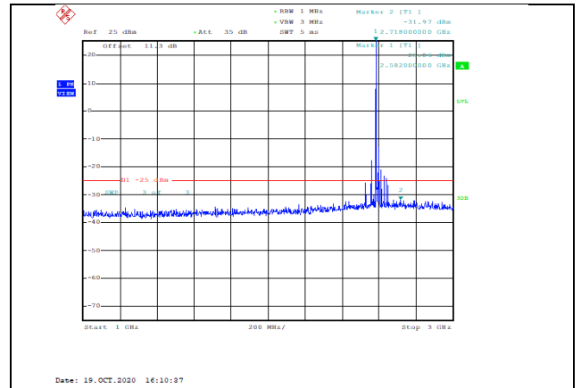
Band41-20MHz-QPSK-40590-1RB#0- Range2:1000~3000MHz--31.97-PASS
