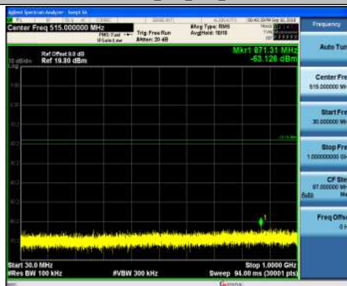
11N20MIMO_Ant1_2457_30~1000
