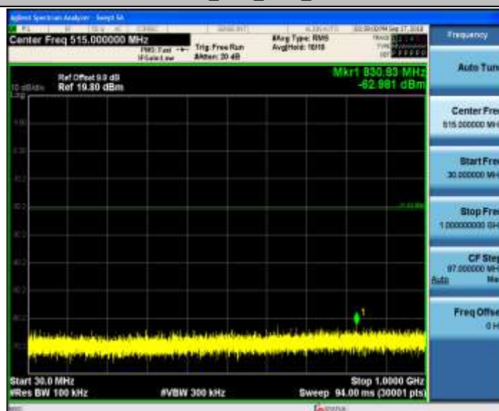
11G-CDD_Ant1_2462_30~1000
