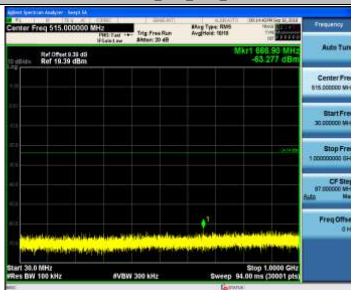
11N40MIMO_Ant2_2447_30~1000
