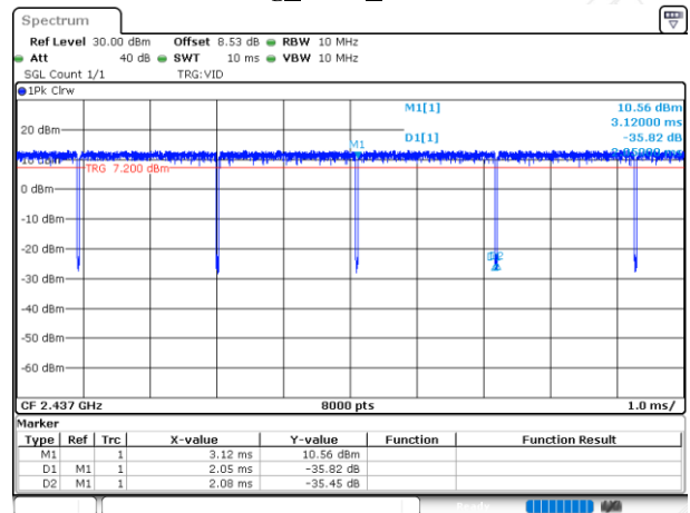
802.11g_Ant1_2437MHz
