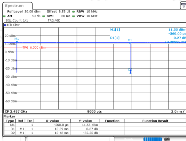
802.11b_Ant1_2437MHz
