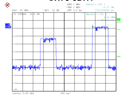
CH78-3DH1
