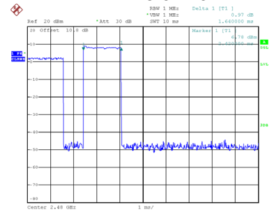
CH78-3DH3
