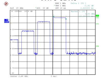
CH78-3DH5
