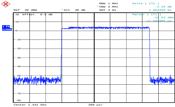
\pi/4 -DQPSK_Hopping_2DH3 1.664ms
