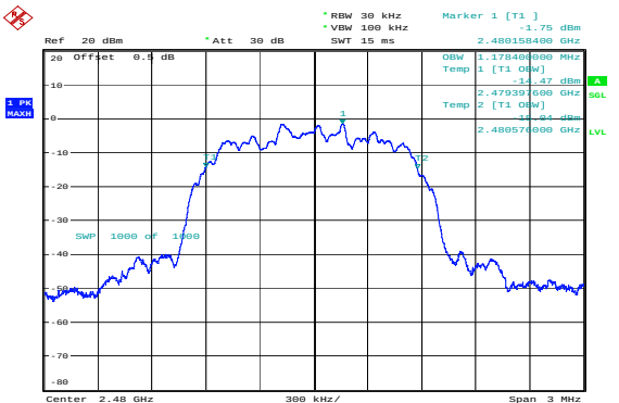
\pi/4 -DQPSK_High 1.178MHz
