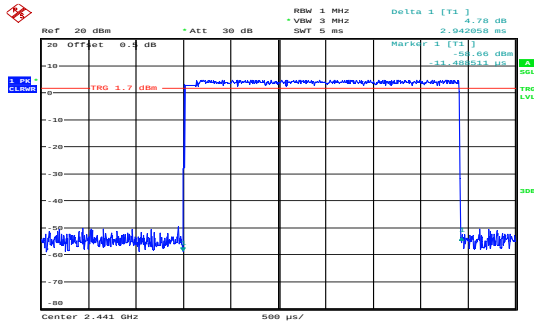
\pi/4 -DQPSK_Hopping_2DH5 2.942ms
