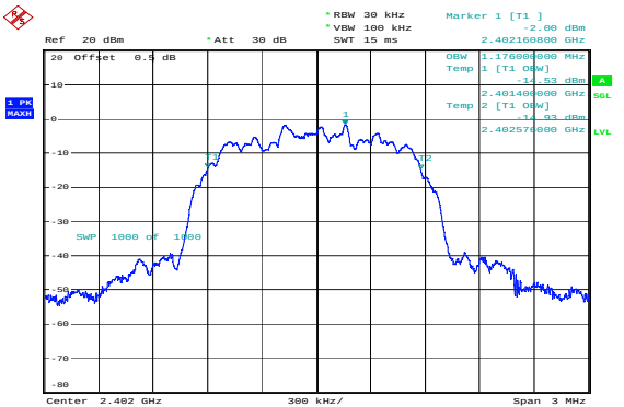
\pi/4 -DQPSK_Low 1.176MHz
