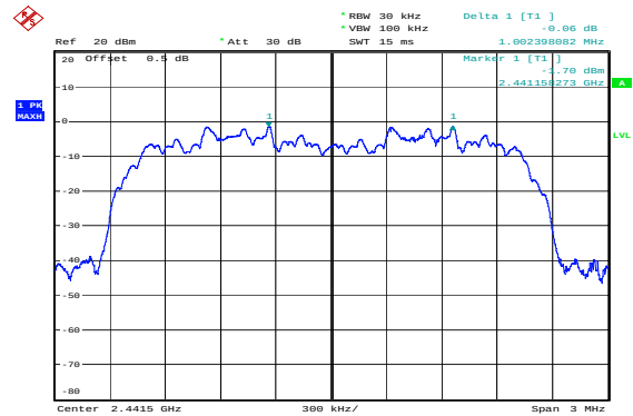
\pi/4 -DQPSK_Middle 1.002MHz
