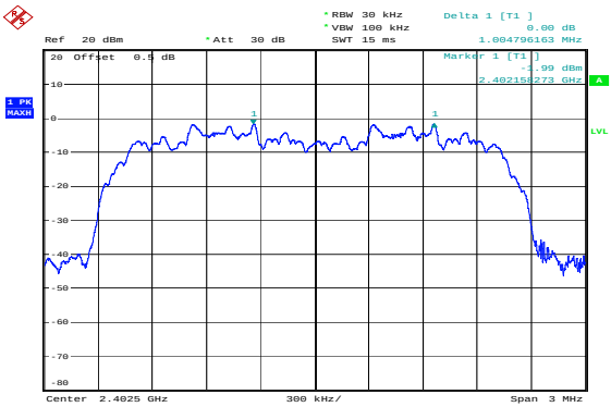
\pi/4 -DQPSK_Low 1.005MHz
