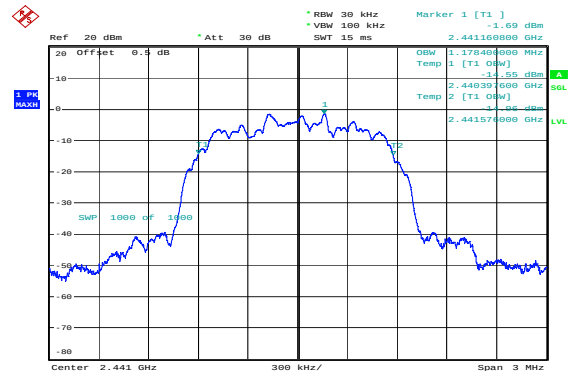
\pi/4 -DQPSK_Middle 1.178MHz
