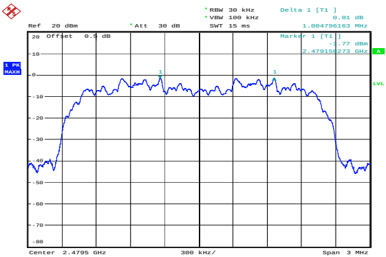
\pi/4 -DQPSK_High 1.005MHz
