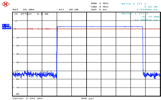
GFSK_Hopping_DH5 2.942ms
