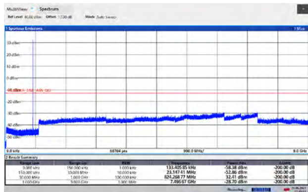
GSM 850 CH-Middle 9kHz ~ 9GHz
