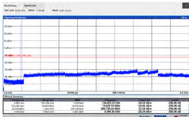
GSM 850 CH-High 9kHz ~ 9GHz
