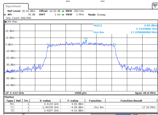
802.11n20_2412MHz_Chain 1
