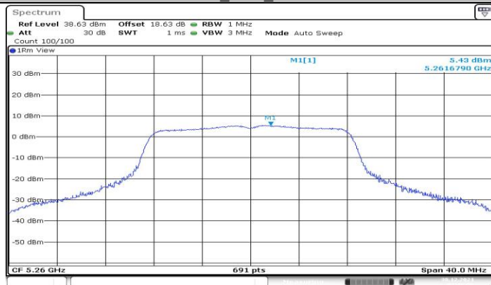
11A_Ant1_5260
