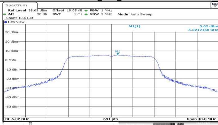
11A_Ant1_5320
