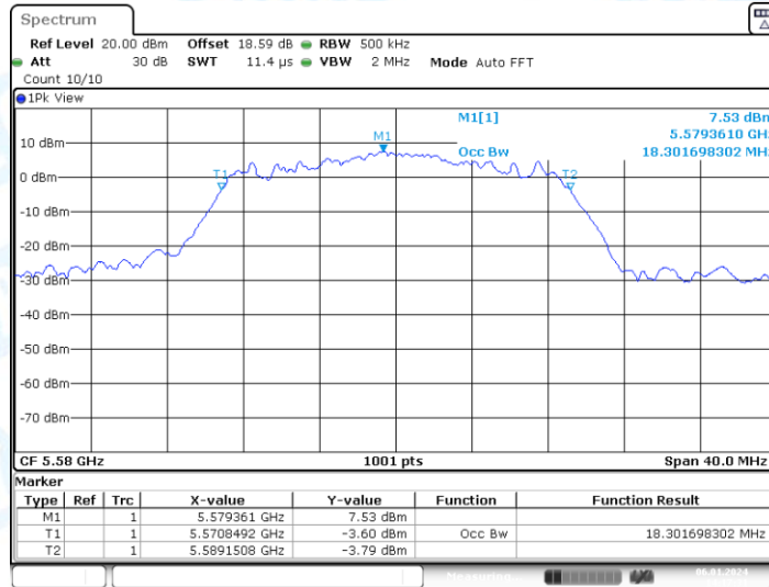
11N20-CDD_Ant2_5580
