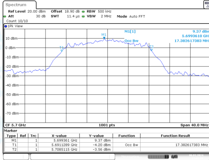
11A-CDD_Ant2_5700
