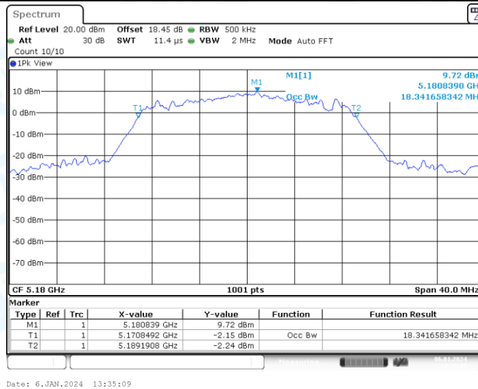
11N20-CDD_Ant2_5180
