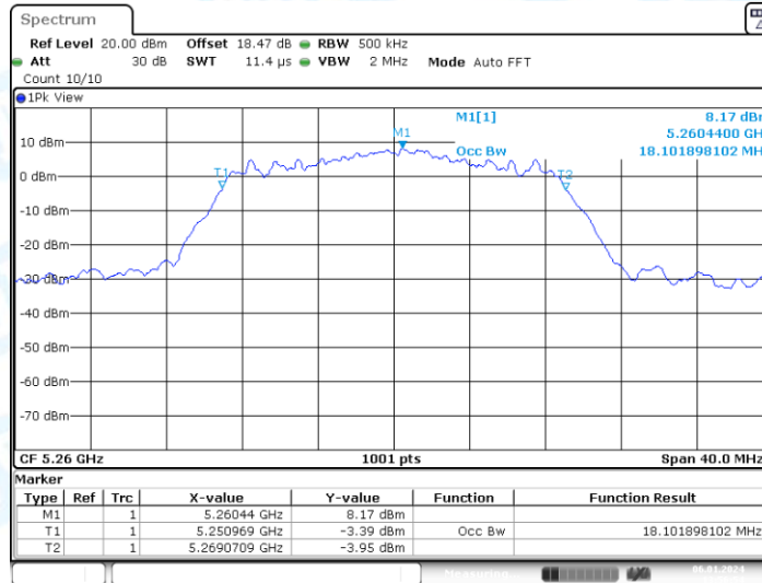
11N20-CDD_Ant1_5260
