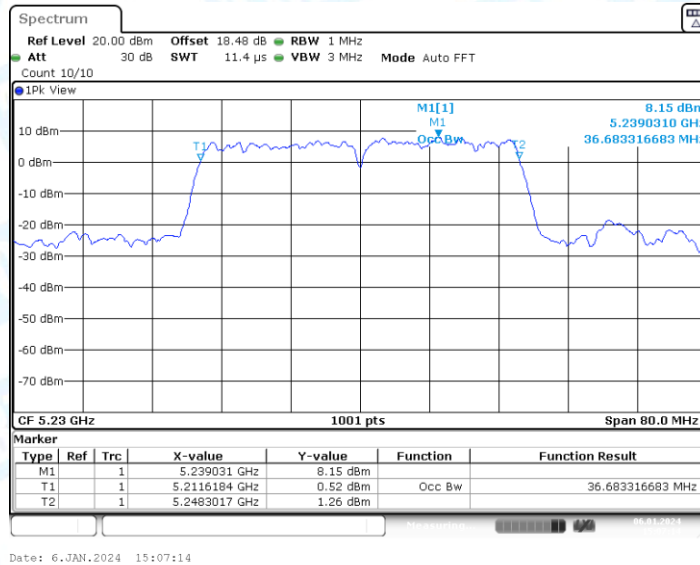
11N40-CDD_Ant2_5230
