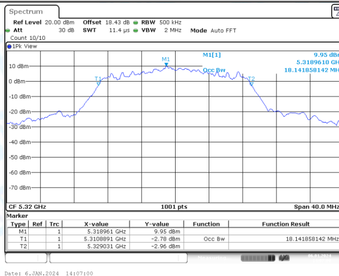
11N20-CDD_Ant2_5320
