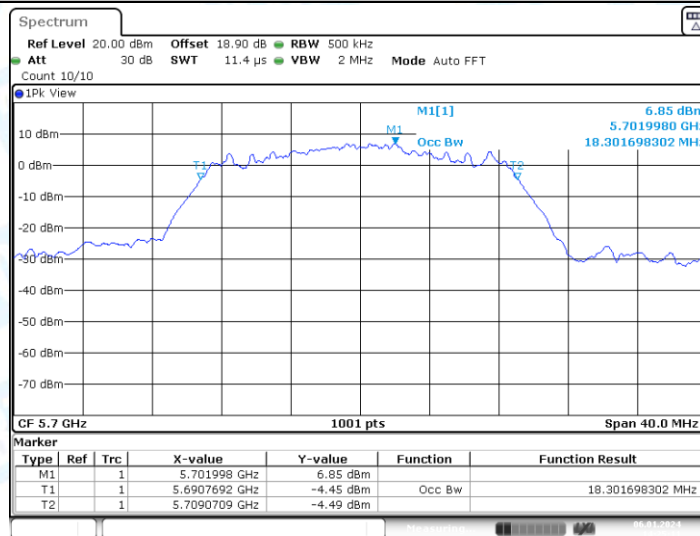
11N20-CDD_Ant1_5700
