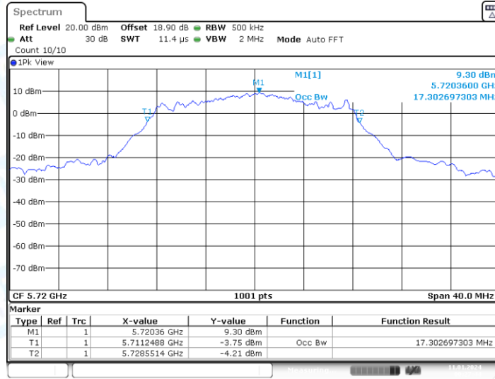
11A-CDD_Ant1_5720
