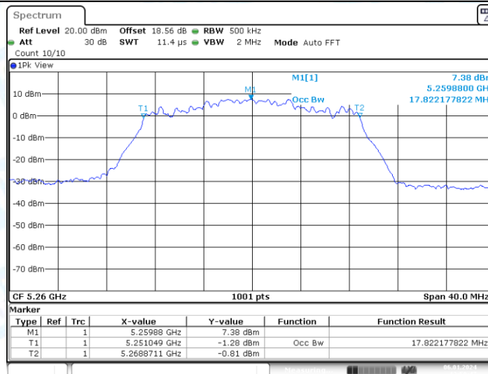
11N20-CDD_Ant2_5260
