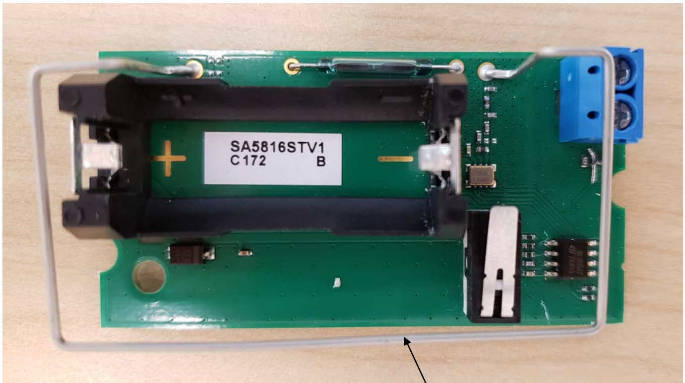
PCB TOP
