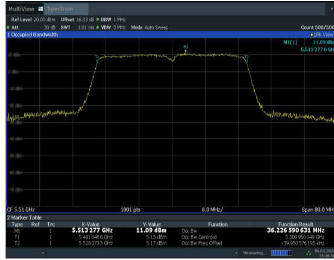
11AC40MIMO_ANT10_5510
