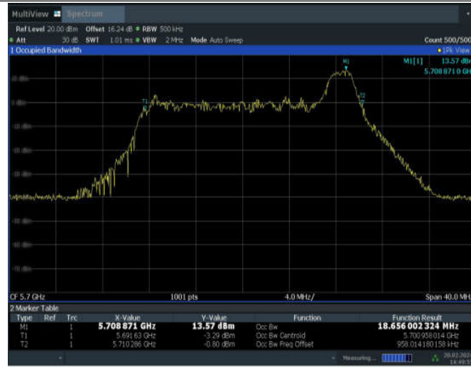
11AX20MIMO_ANT7_5700_26Tone_RU8
