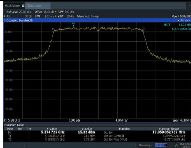
11AX20SISO_ANT10_5280
