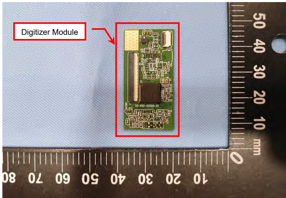
EUT Photo (88)
