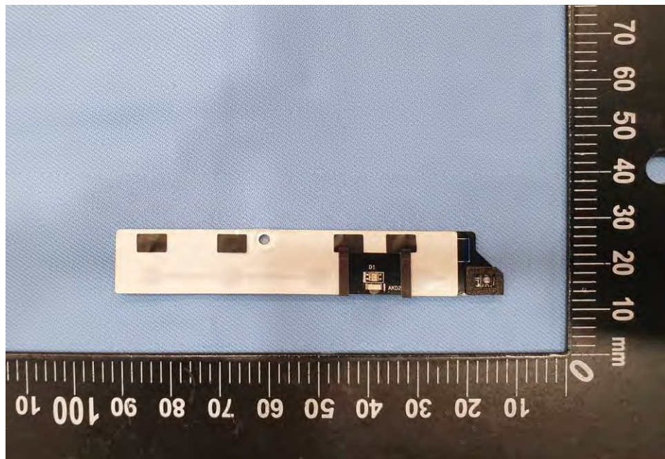
EUT Photo (82)
