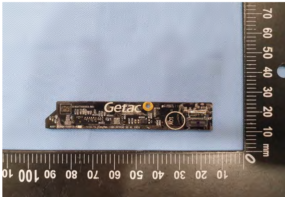
EUT Photo (84)
