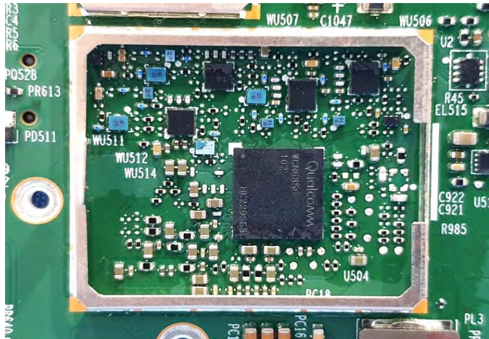
EUT Photo (50)
