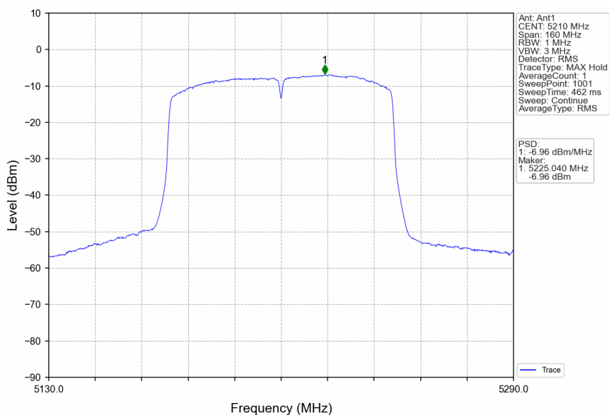
802.11ac(VHT80)_MCH_5210MHz_Ant1_NTNV
