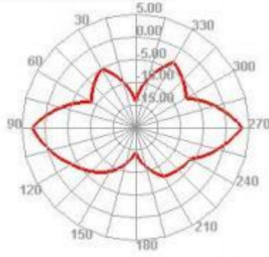
2400.000MHz E1
