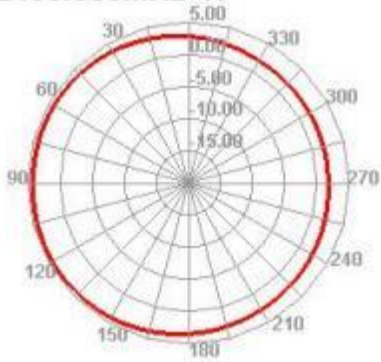
2400.000MHz H
