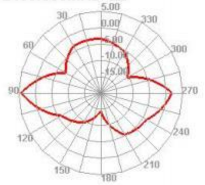
2400.000MHz E2
