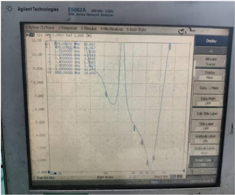
无源驻波图
