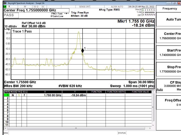
Band Edge_Band4_15MHz_QPSK_RB1_74_CH20325
