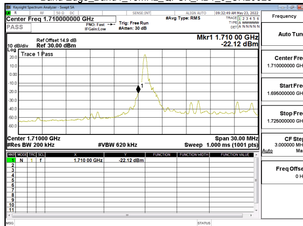
Band Edge_Band4_15MHz_QPSK_RB1_74_CH20325
