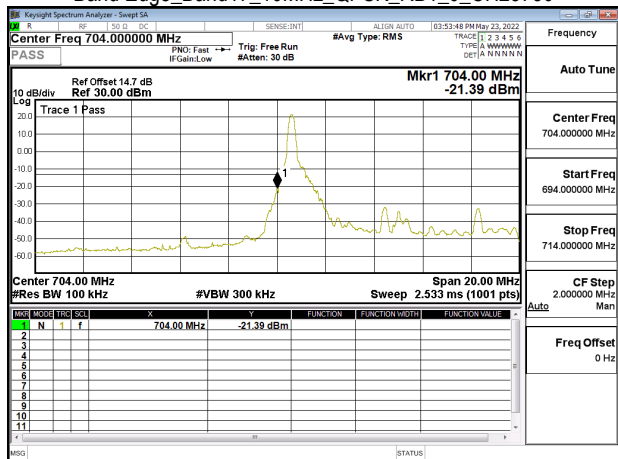
Band Edge_Band17_10MHz_QPSK_RB1_49_CH23800
