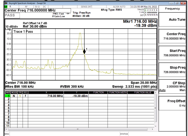
Band Edge_Band12_10MHz_QPSK_RB1_49_CH23130
