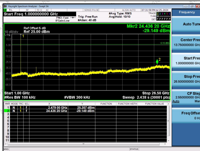
2.4G-Ant1-2479.4-1000~26500-PASS
