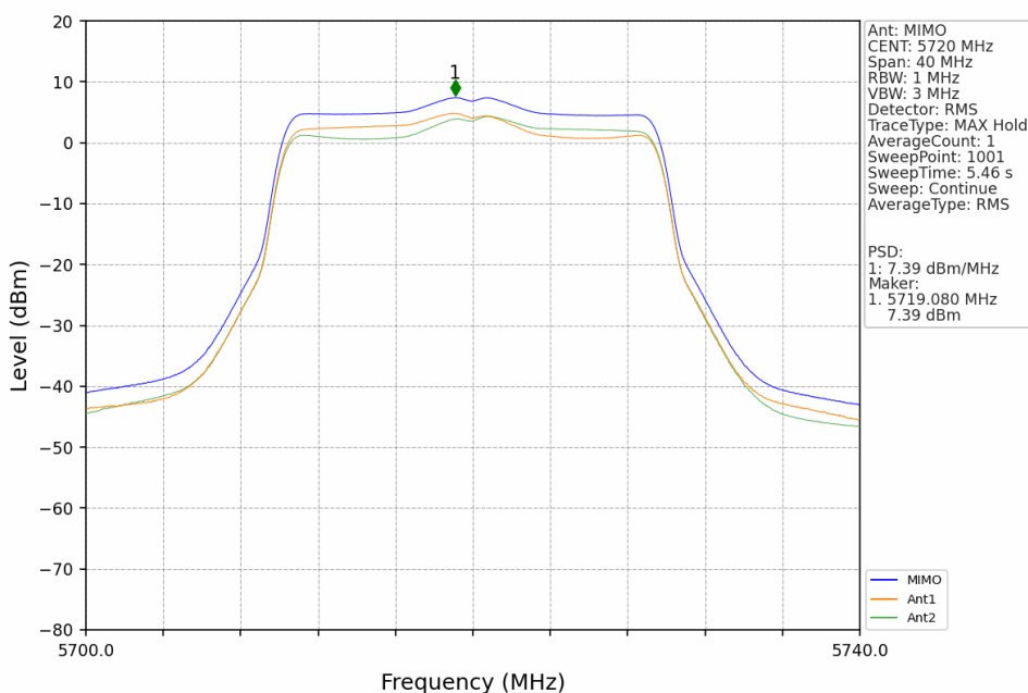
802.11be(EHT20)_HCH_5720MHz_SU_MIMO_NTNV
