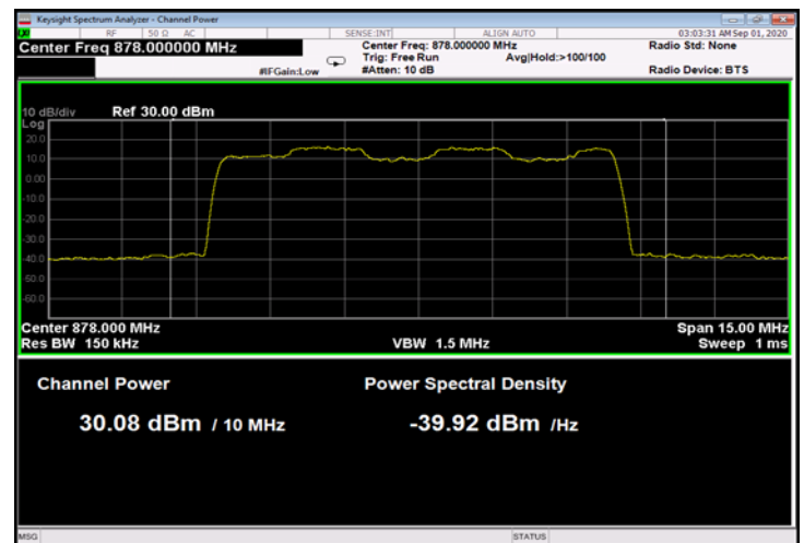
Figure 19: 16QAM 10MHz B.W.; 878.0MHz, 60kHz
