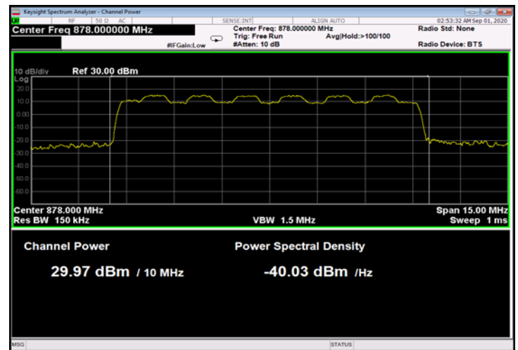
Figure 17: 16QAM 10MHz B.W.; 878.0MHz, 15kHz
