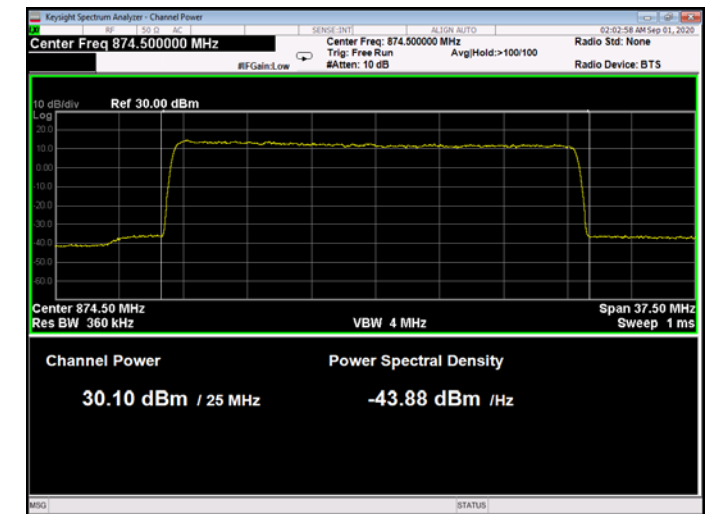
Figure 84: 64QAM 25MHz B.W.; 874.5MHz, 30kHz
