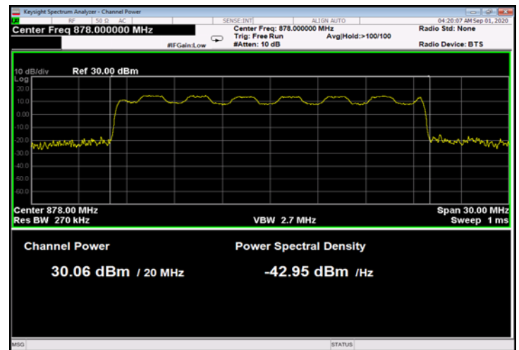
Figure 35: 16QAM 20MHz B.W.; 878.0MHz, 15kHz
