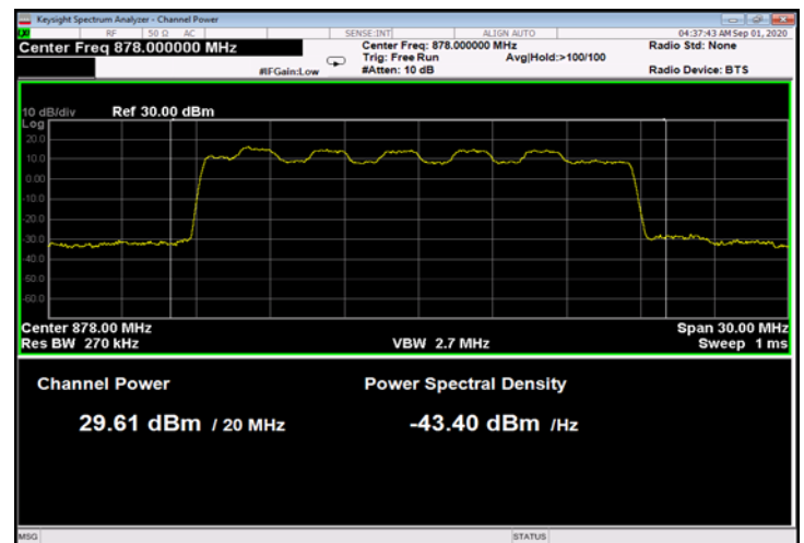
Figure 37: 16QAM 20MHz B.W.; 878.0MHz, 60kHz
