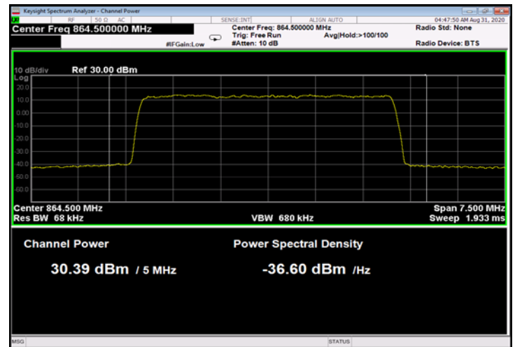
Figure 51: 64QAM 5MHz B.W.; 864.5MHz, 30kHz
