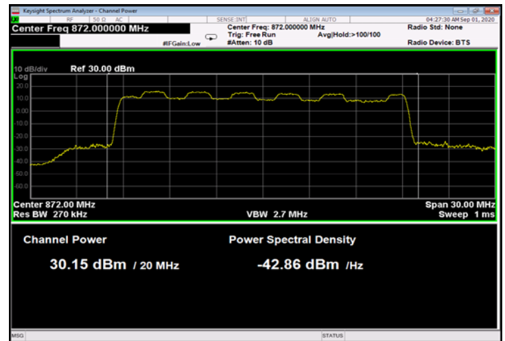
Figure 33: 16QAM 20MHz B.W.; 872.0MHz, 30kHz
