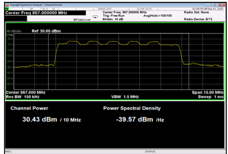
Figure 15: 16QAM 10MHz B.W.; 867.0MHz, 30kHz
