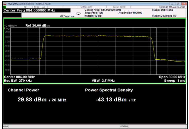
Figure 81: 64QAM 20MHz B.W.; 884.0MHz, 30kHz
