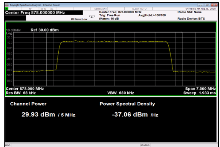
Figure 53: 64QAM 5MHz B.W.; 878.0MHz, 30kHz
