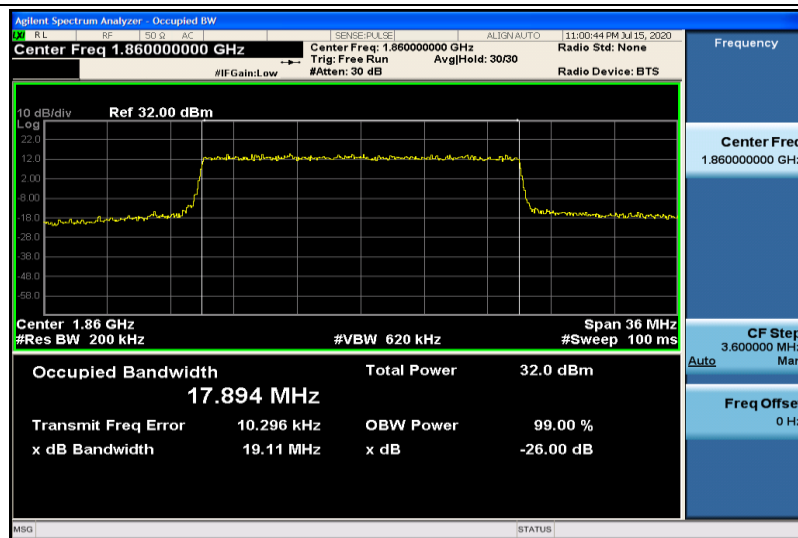
Band2-20MHz-QPSK-18700-100RB#0-17.894
