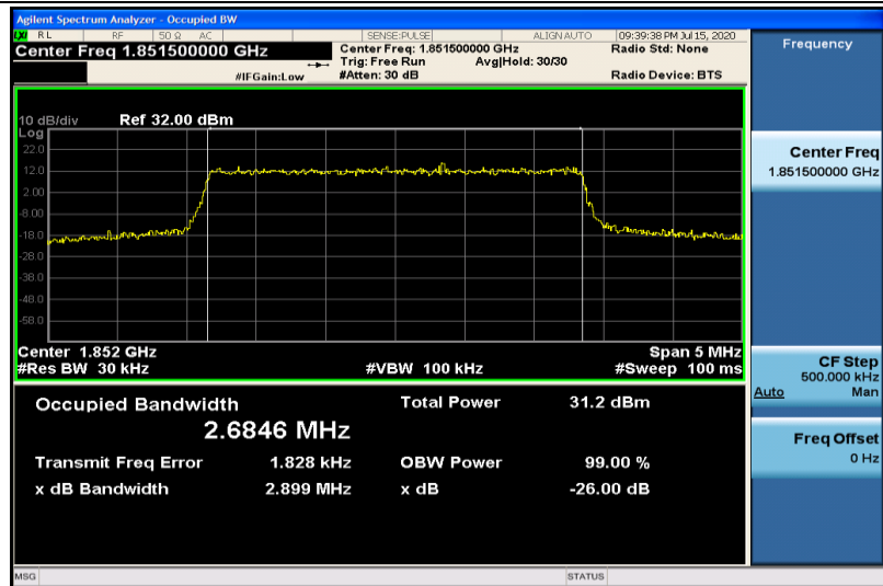
Band2-3MHz-QPSK-18615-15RB#0-2.6846
