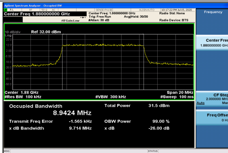
Band2-10MHz-QPSK-18900-50RB#0-8.9424
