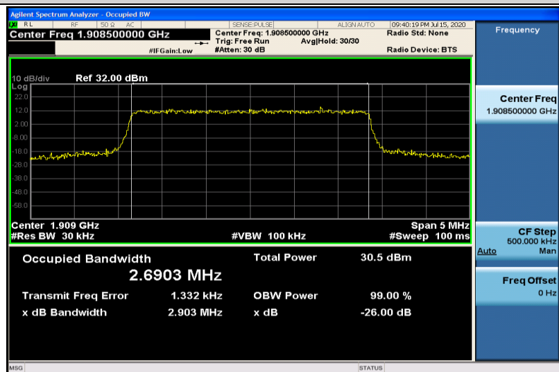
Band2-3MHz-QPSK-19185-15RB#0-2.6903
