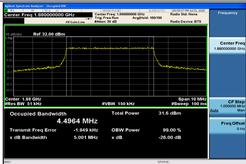
Band2-5MHz-QPSK-18900-25RB#0-4.4964
