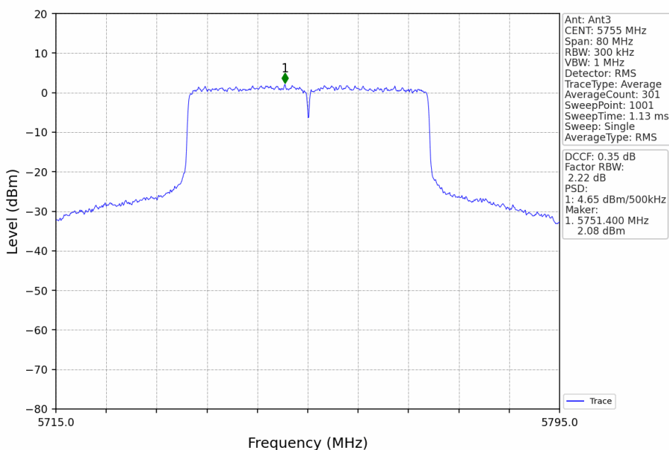
802.11ax(HEW40)_LCH_5755MHz_RU484_Left_Ant3_NTNV
