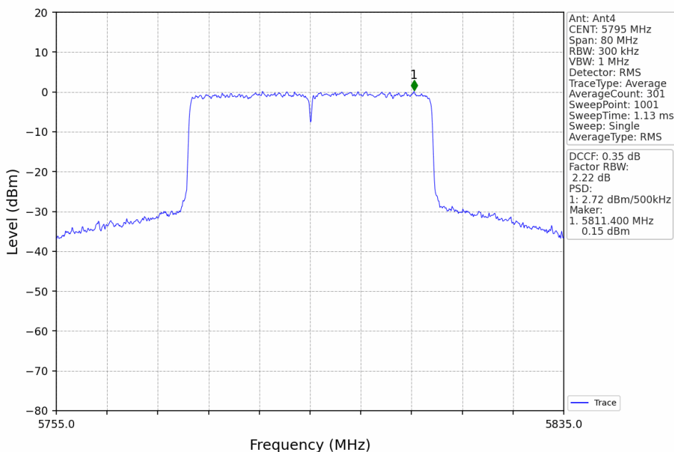
802.11ax(HEW40)_HCH_5795MHz_RU484_Left_Ant4_NTNV
