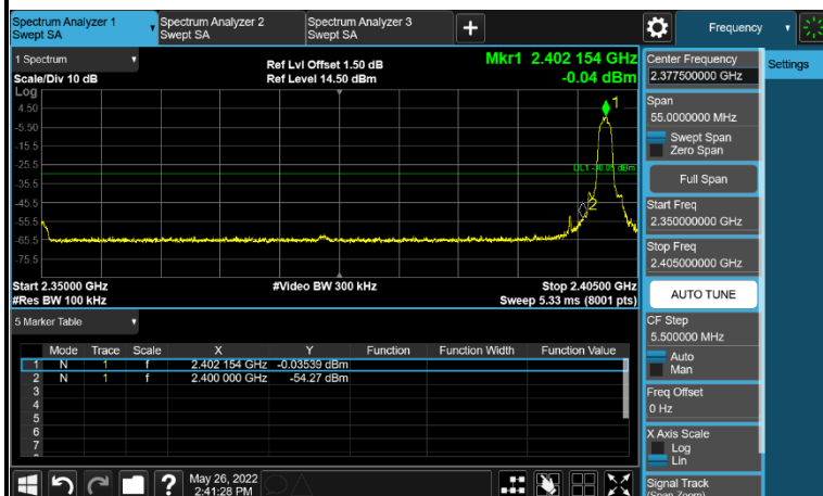
Mode 2 CH00(2402MHz)
