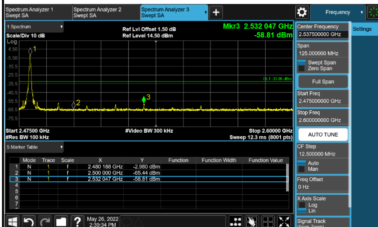
Mode 1 CH78(2480MHz)
