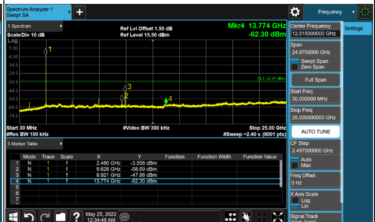
Mode 1 CH78(2480MHz)
