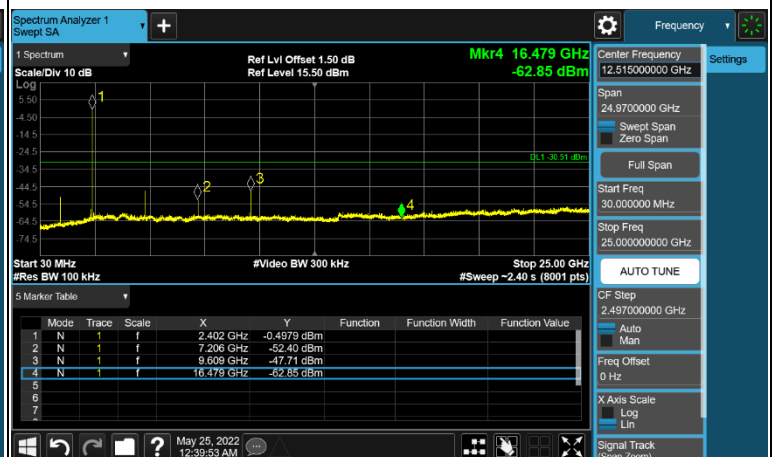
Mode 2 CH00(2402MHz)
