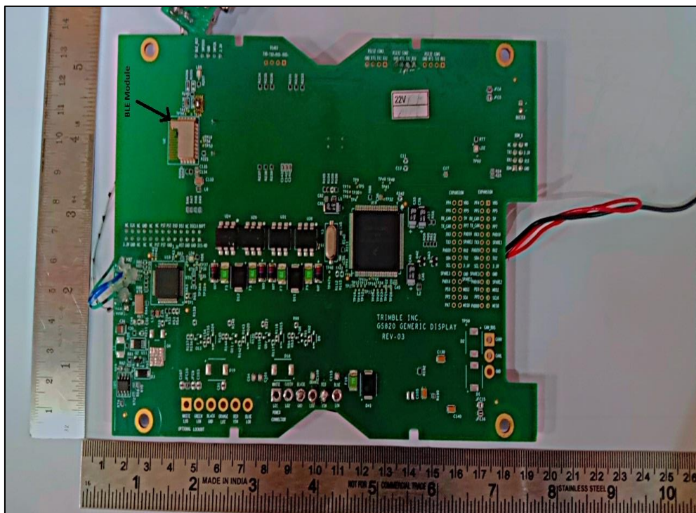
Figure 4: BLE Module Location
