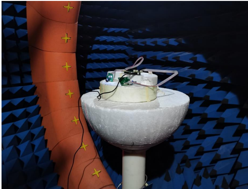
有源测试
