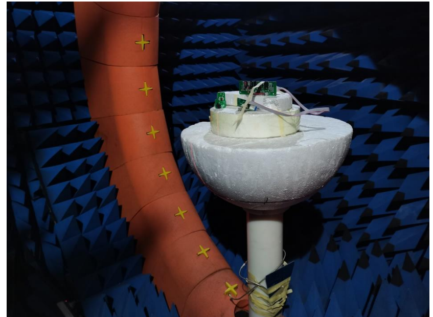
无源测试
