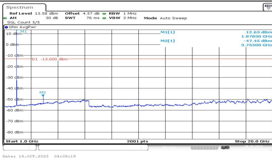
Band25-10MHz-QPSK-26365-1RB#0-Range4:1000~20000MHz-PASS
