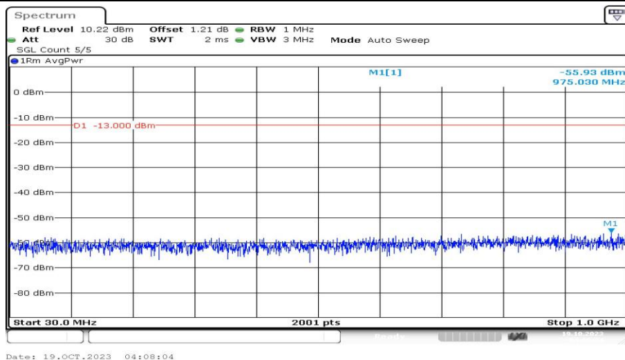
Band25-10MHz-QPSK-26365-1RB#0-Range3:30~1000MHz-PASS
