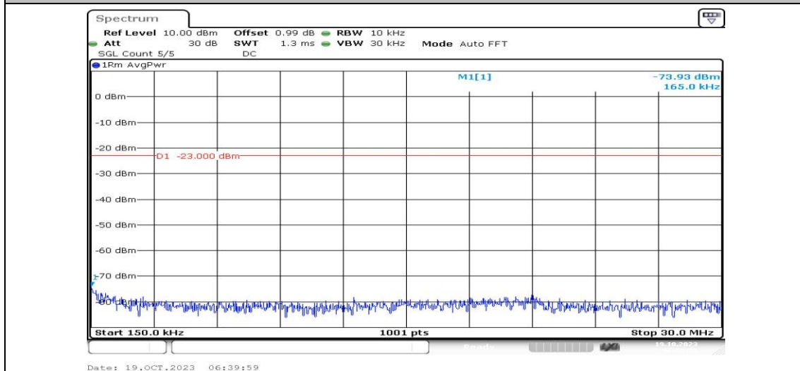
Band25-20MHz-16QAM-26590-1RB#0-Range2:0.15~30MHz-PASS
