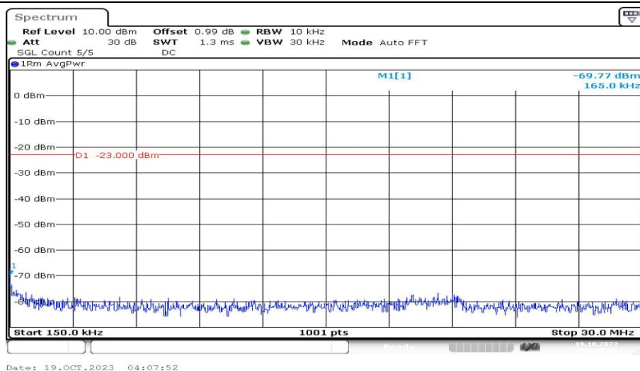
Band25-10MHz-QPSK-26365-1RB#0-Range2:0.15~30MHz-PASS
