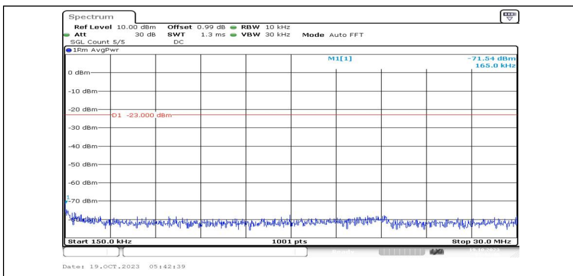
Band25-10MHz-16QAM-26365-1RB#0-Range2:0.15~30MHz-PASS
