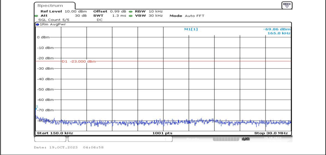
Band25-10MHz-QPSK-26090-1RB#0-Range2:0.15~30MHz-PASS
