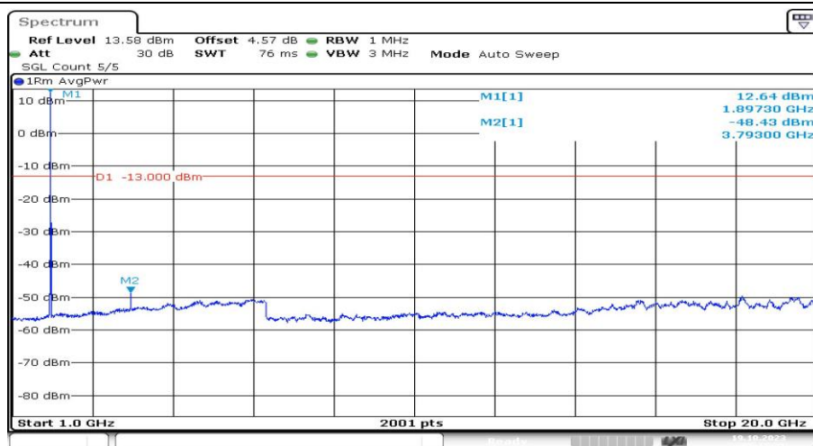
Band25-20MHz-QPSK-26590-1RB#0-Range4:1000~20000MHz-PASS
