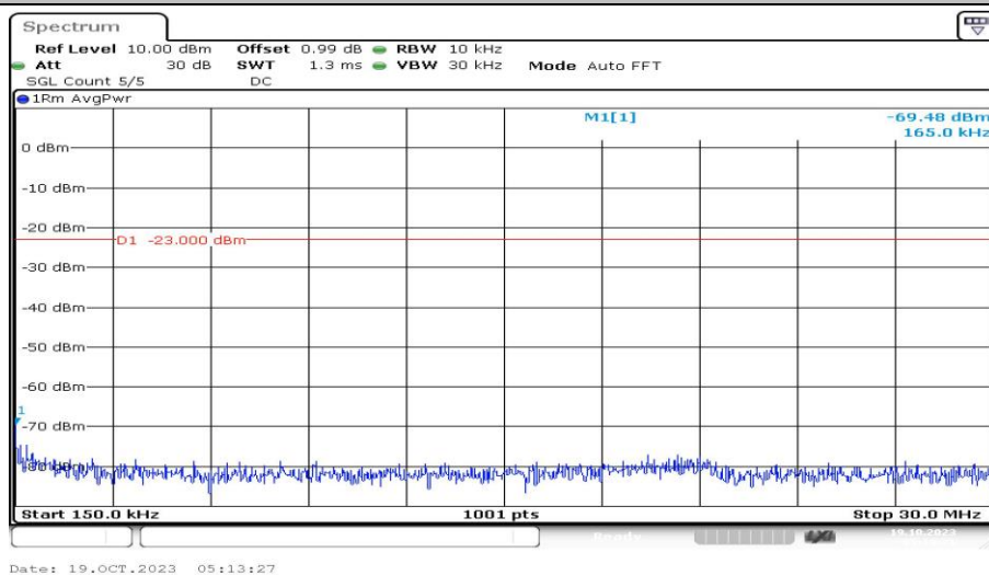
Band25-20MHz-QPSK-26140-1RB#0-Range2:0.15~30MHz-PASS
