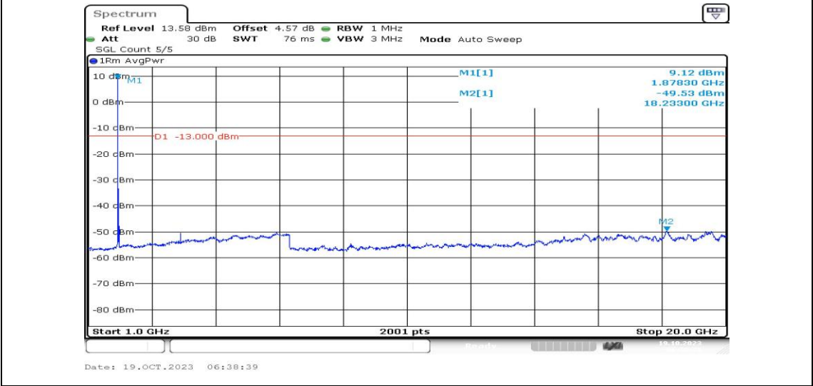
Band25-20MHz-16QAM-26365-1RB#0-Range4:1000~20000MHz-PASS
