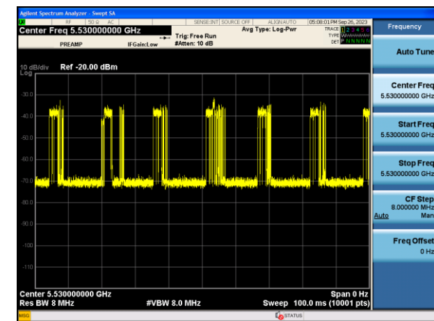
802.11ax-HE80 (5530MHz)
